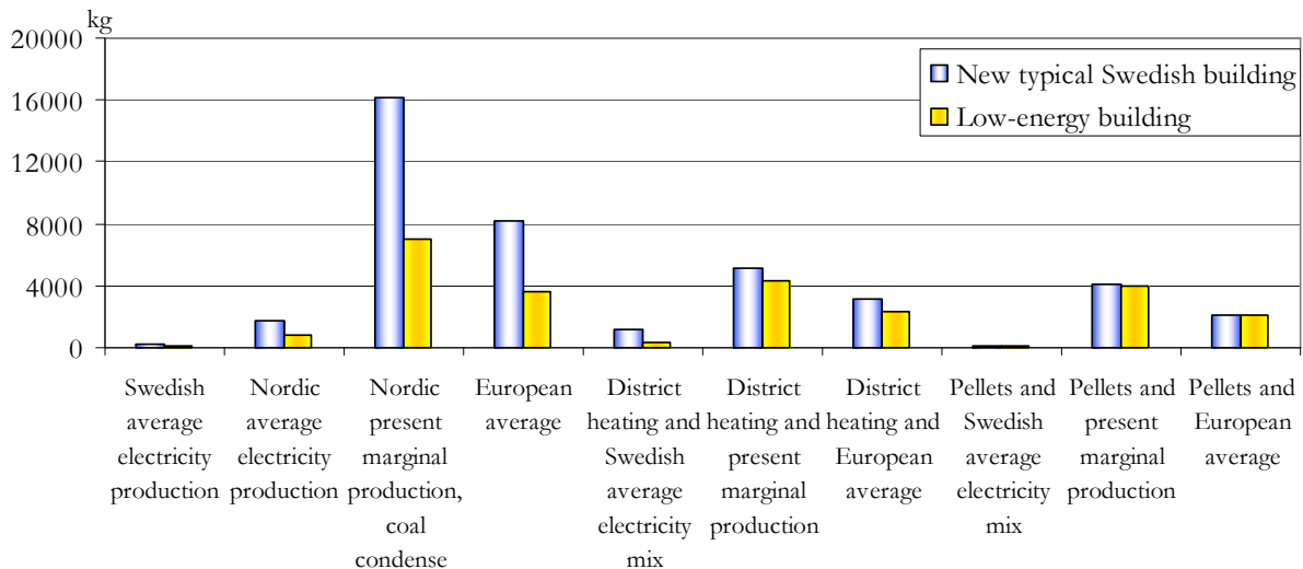
Figur 1. Koldioxidutsläpp från ett lågenergihus (62,5 kWh/m 2 ,år) och ett nytt svenskt standardhus (142 kWh/m 2 ,år) [Karlsson 2006].
