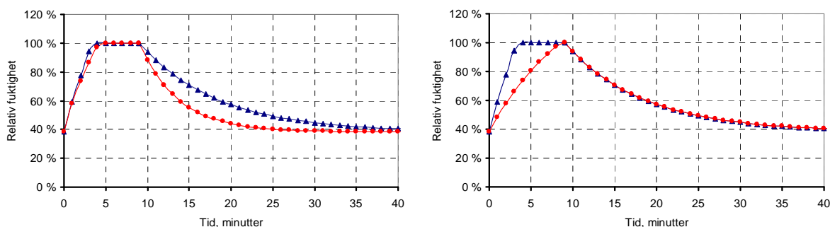
Figur 2. Beregnet relativ fuktighet som funksjon av tid i badrom ved dusjing. Rommets areal er 3.7 m 2 . I venstre del av figuren viser kurve med trekantede 15 l/s i lufttilførsel og kurve med prikkede 30 l/s. I høyre del av figuren viser kurve med trekantede normal fukttilførsel og kurve med prikkede representerer halvert fukttilførsel. Lufttilførselen er i dette tilfellet 15 l/s.
