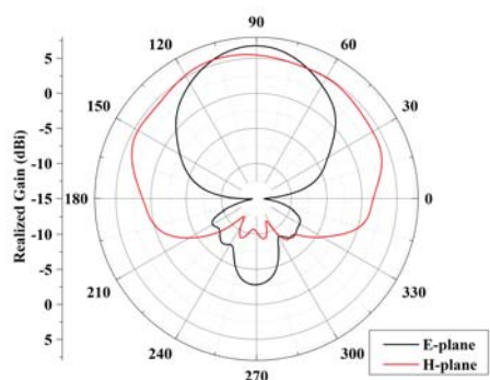
(d) E-plane and H-plane radiation pattern of S band antenna
