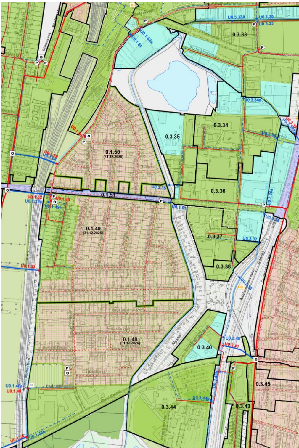
Figur 5.3: Udclip fra Aalborg Kommunes spildevandsplan for Kærby. Grønne områder er separatkloakerede og brune områder er fælleskloakerede. Pumpestationer er angivet med (P) og overløbsbygværker med (O).
