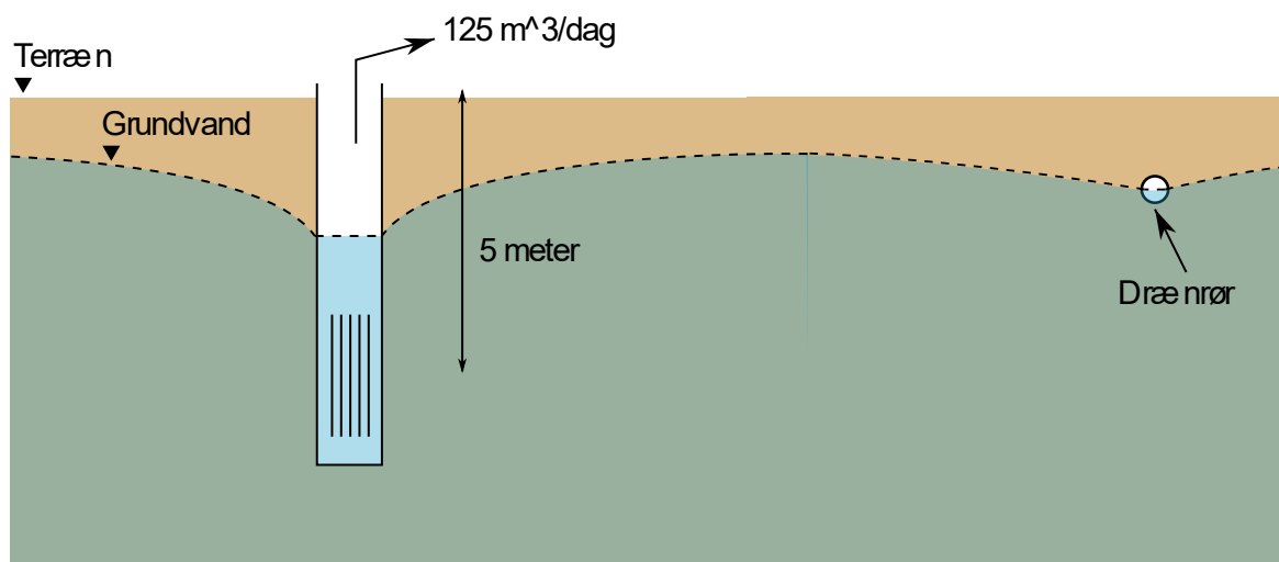
Figur 5.44: Illustration af modelscenariet med en kombination af horisontale og vertikale dræn. De vertikale dræn pumper 125 \text{ m}^3/\text{dag} grundvand fra 5 meters dybde.
