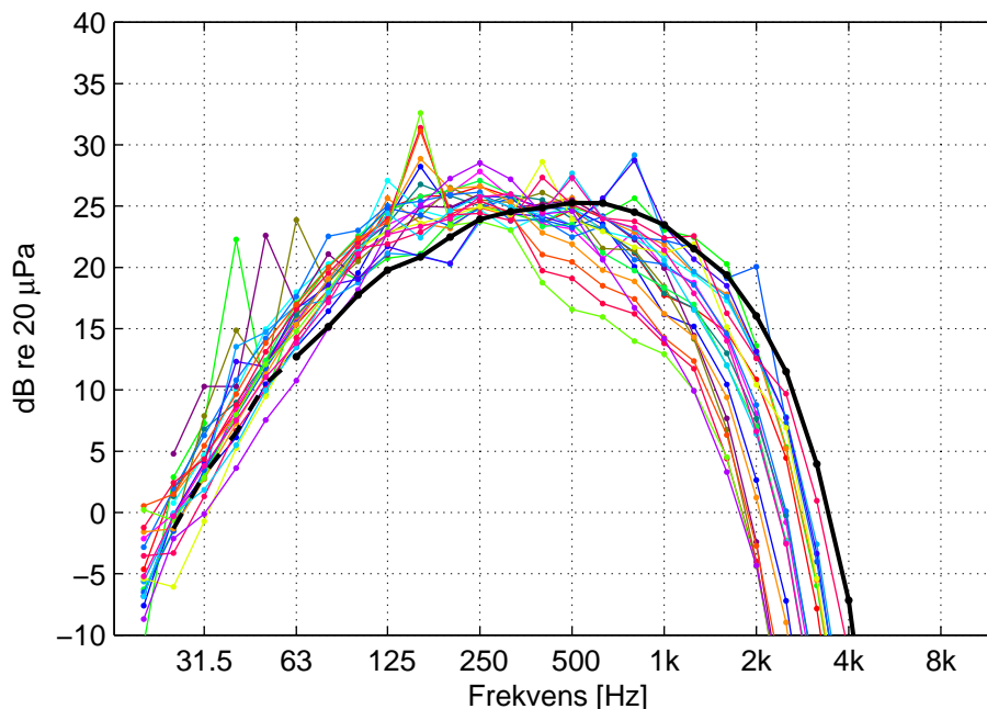
Figur 11. A-vægtet lydtrykniveau i 1/3-oktavbånd ved den afstand, hvor det totale A-vægtede lydtrykniveau er 35 dB (se Tabel 3). Cylindrisk lydudbredelse er antaget fra 200 m. Færgkode for møller som i Figur 5.
