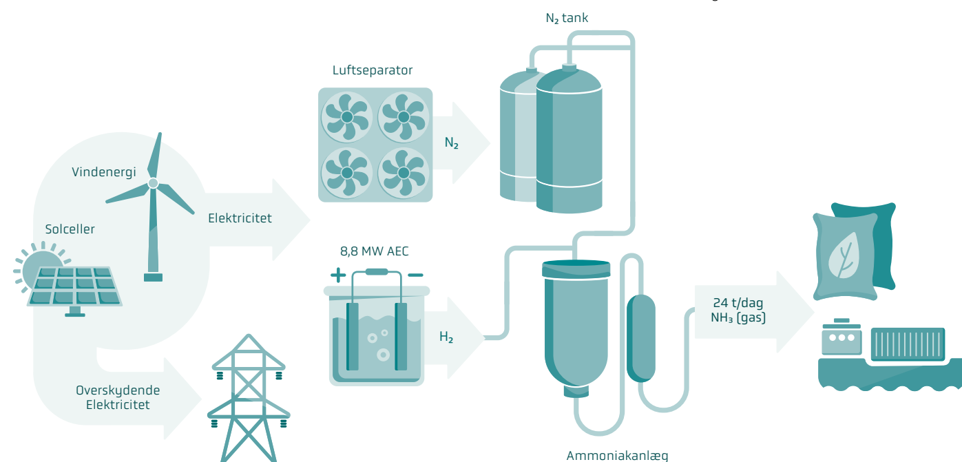
Figur 22: Diagram over REDDAP-projektet. Vedvarende elektricitet fra egne VE-anlæg driver brint- og kvælstofproduktion, som i ammoniak anlægget bliver omdannet til ammoniak (NH 3 ). Overskydende elektricitet bliver solgt til elnettet.
