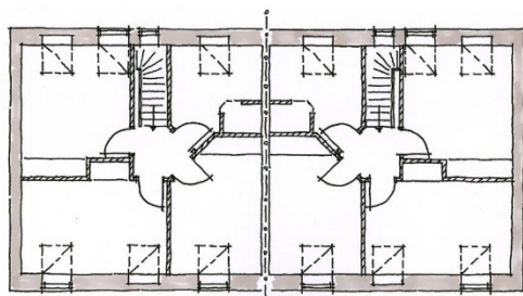
Dobbelthuset 1. sal
