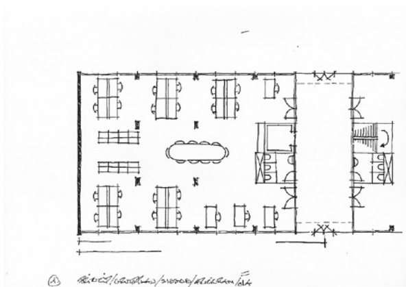
Kontorhuset etageplan
