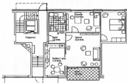
Type 2 st. 3-runs lighted Bruksareal 51,9 kvm.
