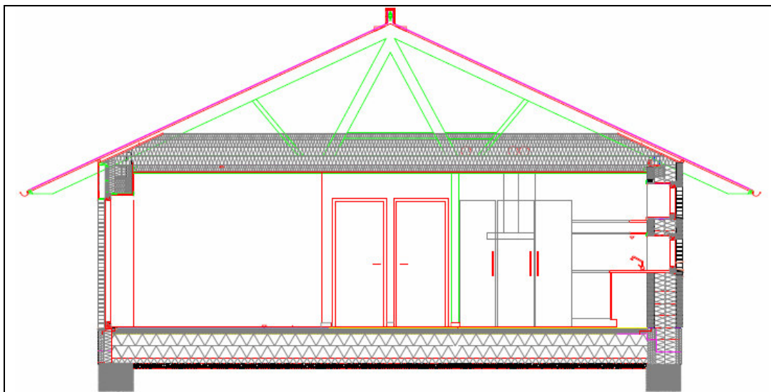
Tværsnit af hus (se tabel med data)
