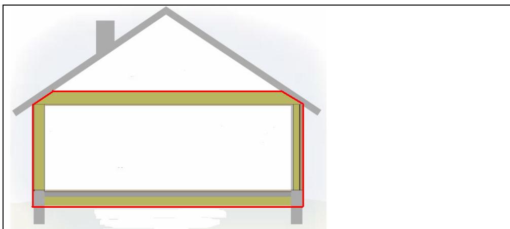
Figur 6: I PHPP bruges udvendige dimensioner overalt ved bestemmelse af transmissionsarealer.
