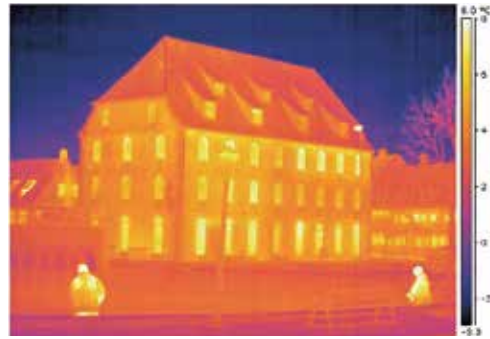
Figur 1. Termografi af bygning med angivelse af kuldebroer
