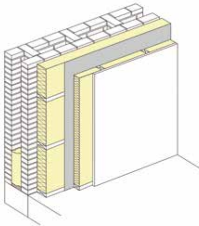
Figur 2. Udsnit i hulmur i tegl med faste bindere og indvendig efterisolering. Dampspærren sidder mellem isoleringslagene og evt. installationer føres i isoleringslaget mod rummet. For at sikre tæthed skal alle samlinger og tilslutninger mod væg, loft og andre vægge være klæbet og have fast underlag.
