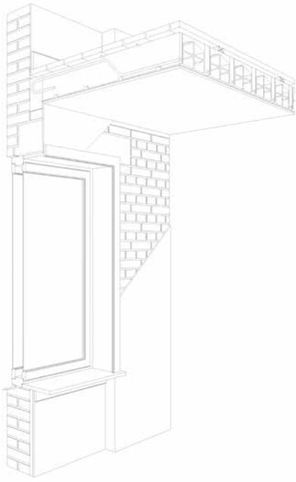
Figur 3. Udsnit af dæk / facade.
