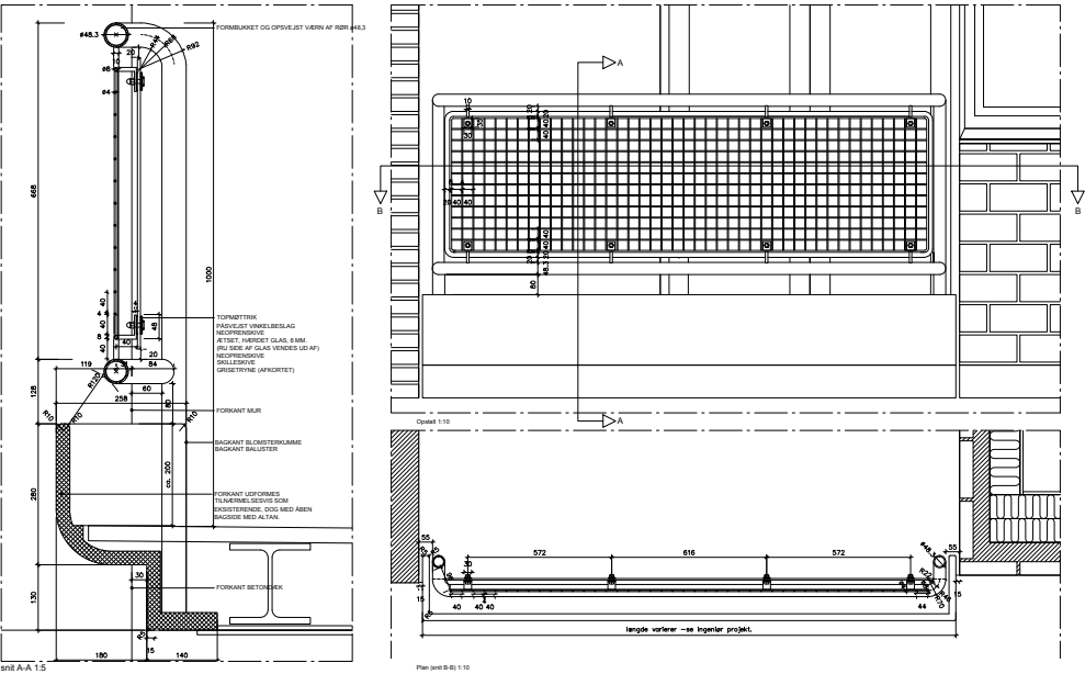
Tegningen viser de nye værn, blomsterkummer og den nye stålkonstruktion i altanerne, der bærer en del af det eksisterende betondæk samt de nye fiberbetonplader.
