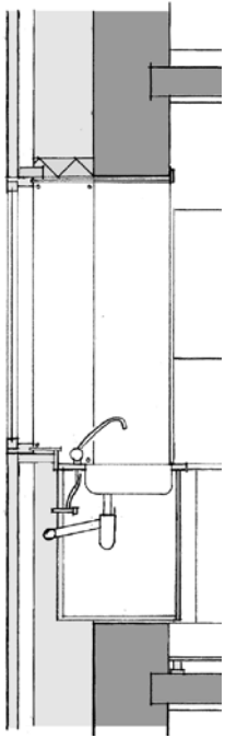
Installationskarnappen indeholder de lodrette føringsveje for vand, afløb og ventilation til badeværelset.
