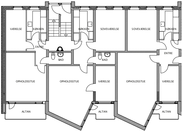
Lejlighed i Sprotoften før placering af elevator og sammenlægning af lejligheder.
