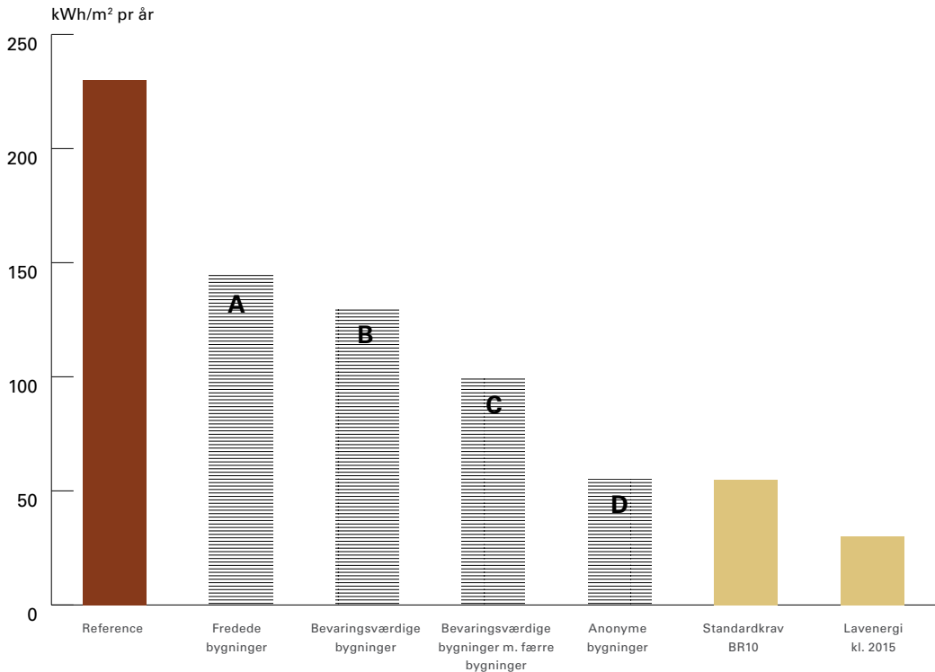
Figur 3. Energiforbrug for referenceejendom og ved energirenovering inden for de fire kulturarvskategorier.
