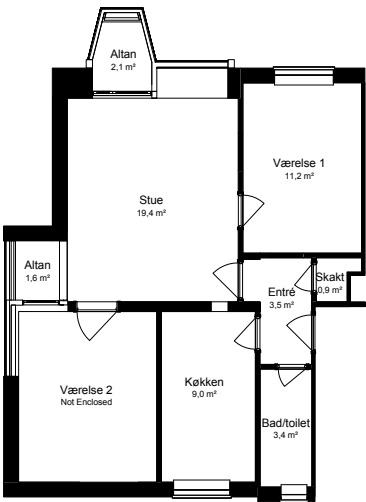
PLAN, EKSISTERENDE FORHOLD
