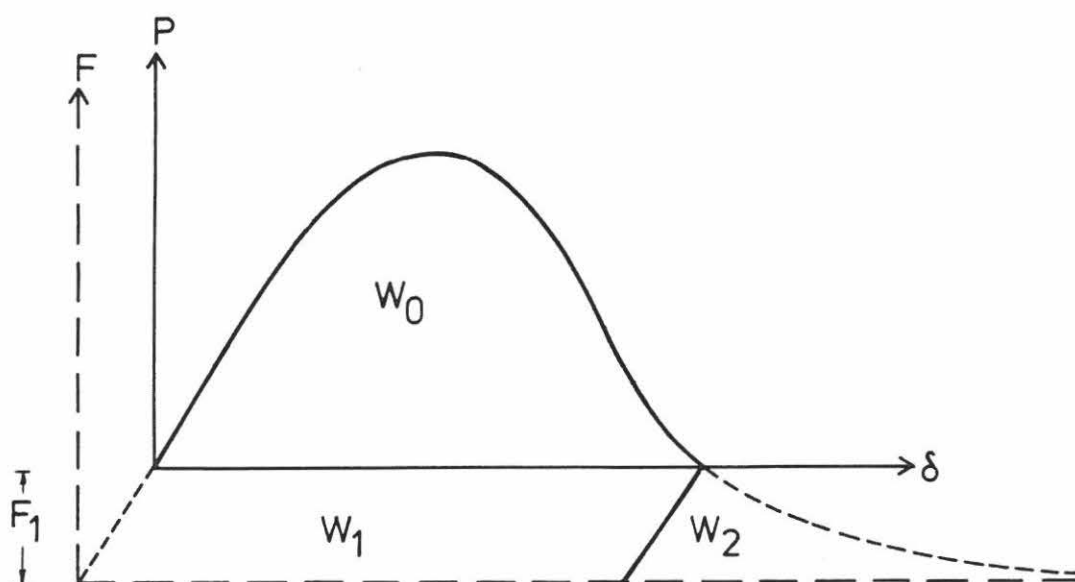
Figur 3. Kraft-deformationskurve.
