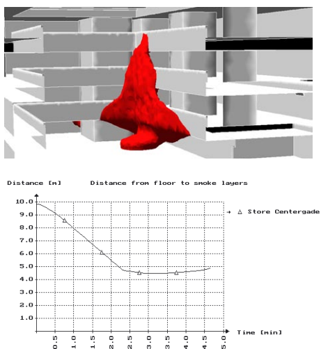
Røgspredning/røglagstykkelsen simuleret med hhv. en CFD-model (top) og en zonemodel (bund) ved en brand i et atrium.
