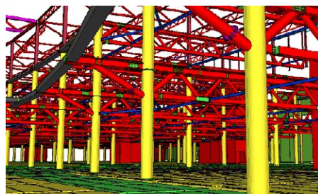
Eksempel på konstruktionsmodel udarbejdet i Tekla
