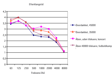
Beregnet middel-efterklangstid i Arena
