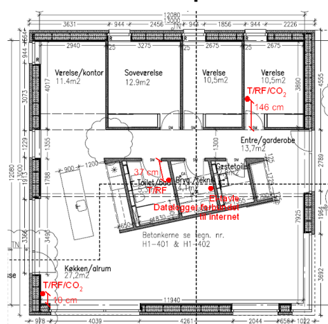
Figur 1. Grundplan
