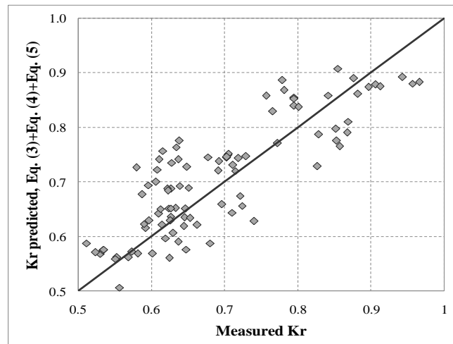
Figura 7. Coefficiente di riflessione misurato e stimato mediante la formula di Zanuttigh & Van der Meer (2008) con l'inclusione della eq. (6) e (7).
