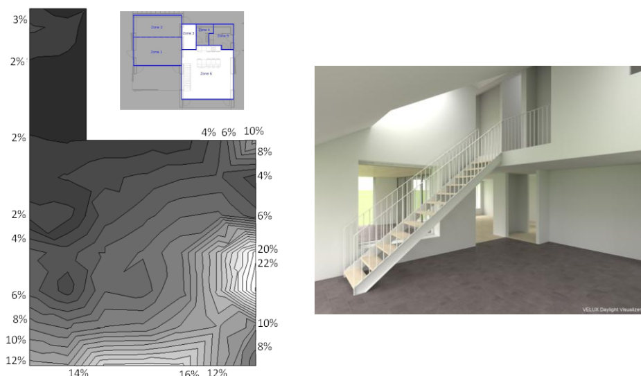
Figur 6.3. Dagslysmålinger foretaget i "Bolig for Livet" i husets alrum. [VKR, 2010]
