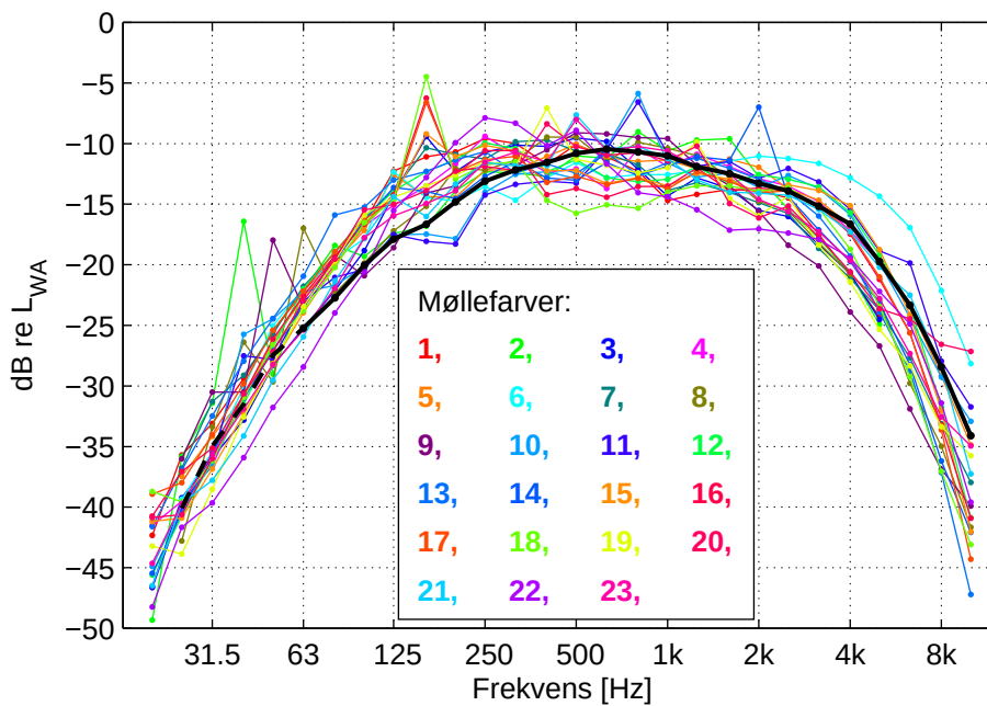
Figur 5. Normerede A-vægtede lydeffektniveauer i 1/3-oktavbånd. Gennemsnit af 39 møller \leq 2 MW (tyk sort linje) og 23 individuelle møller > 2 MW.
