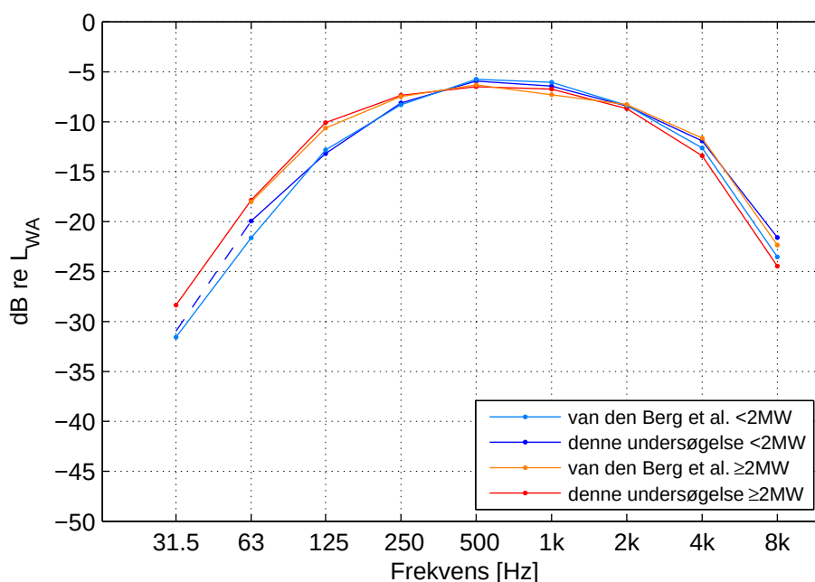
Figur 15. Normeret A-vægtet lydeffektniveau i oktavbånd, gennemsnit for to grupper af møller: < 2 MW og ≥ 2 MW og fra to undersøgelser: van den Berg et al. [75, Appendix D] og denne undersøgelse.
