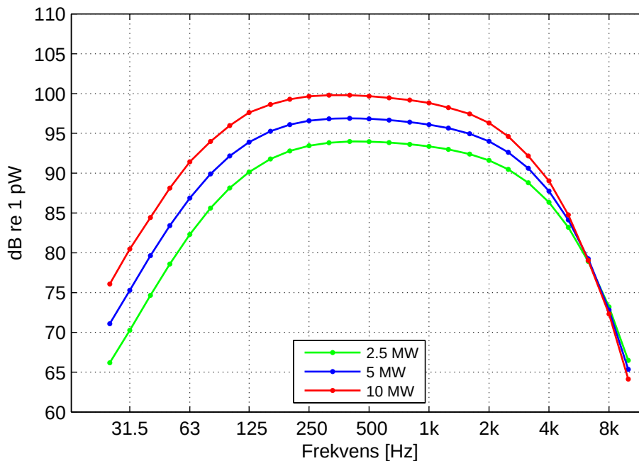
Figur 19. Estimerede A-vægtede lydeffektniveauer i 1/3 oktavbånd for møller omkring 2,5, 5 og 10 MW. Værdier og forudsætninger fra Tabel 3.
