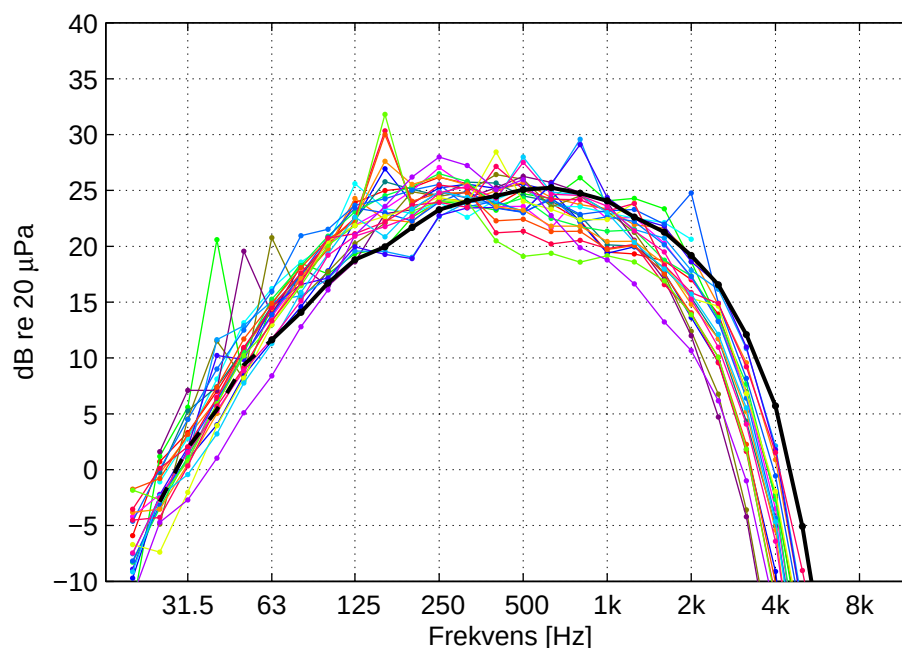
Figur 9. A-vægtet lydtrykniveau i 1/3-oktavnband ved den afstand fra hver enkelt mølle, hvor det totale A-vægtede lydtrykniveau er 35 dB (se Tabel 1). Gennemsnit af 39 møller \leq 2 MW (tyk sort linje) og 23 individuelle møller > 2 MW. Farvekode for møller som i Figur 5.
