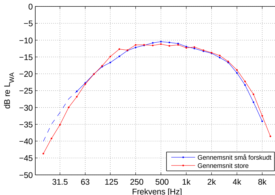
Figur 17. Normerede A-vægtede lydeffektniveauer for 1/3-oktavbånd. Gennemsnit for to grupper af møller; \leq 2 MW og > 2 MW, gruppen af små møller forskudt 1/3 oktav nedad i frekvens.
