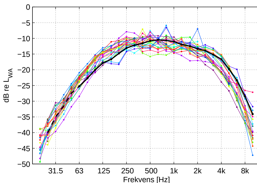
Figur 16. Normerede A-vægtede lydeffektniveauer givet i 1/3-oktavbånd. Gennemsnit af 39 møller \leq 2 MW (tyk sort linje) og 23 individuelle møller > 2 MW. Toppe i 1/3-oktavbånd under 200 Hz fjernet fra de store møller ved at erstatte niveauet ved toppen med niveauer opnået ved lineær interpolation mellem niveauerne for de to omkringliggende 1/3-oktavbånd. Farvekode for møller som i Figur 5.
