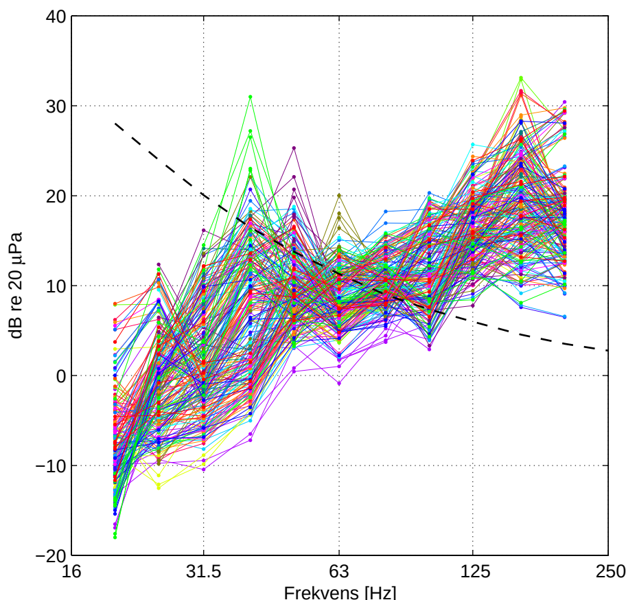
Figur 12. Indendørs A-vægtede lydtrykniveauer for 1/3-oktavbånd i den afstand fra en møllepark, hvor det totale A-vægtede lydtrykniveau udendørs er 44 dB (se Tabel 2). 207 kombinationer af 23 store møller og 9 rum. Stiplet linje er høretærsklen i henhold til ISO 389-7 [29]. Farverne angiver møllen, farvekode som i Figur 5.
