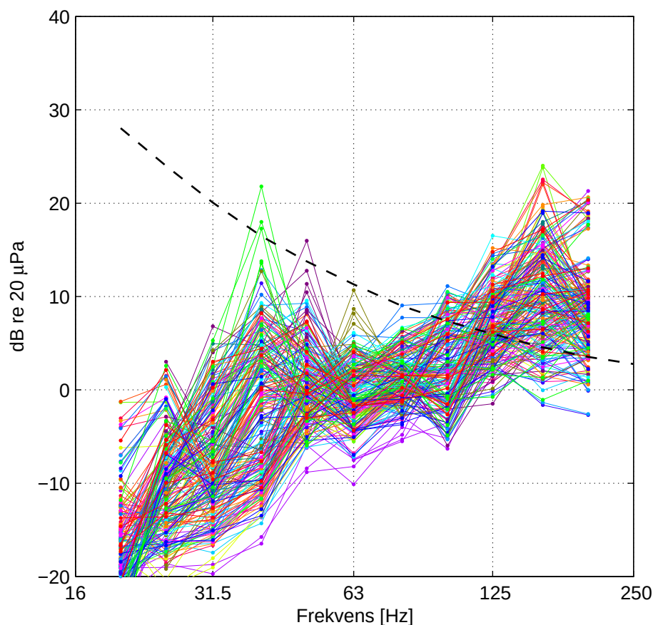
Figur 11. Indendørs A-vægtede lydtrykniveauer for 1/3-oktavbånd i den afstand fra hver enkelt mølle, hvor det totale A-vægtede lydtrykniveau udendørs er 35 dB (se Tabel 1). 207 kombinationer af 23 store møller og 9 rum. Den stiplede linje er høretærsklen i henhold til ISO 389-7 [29]. Farverne angiver møllen, farvekode som i Figur 5.
