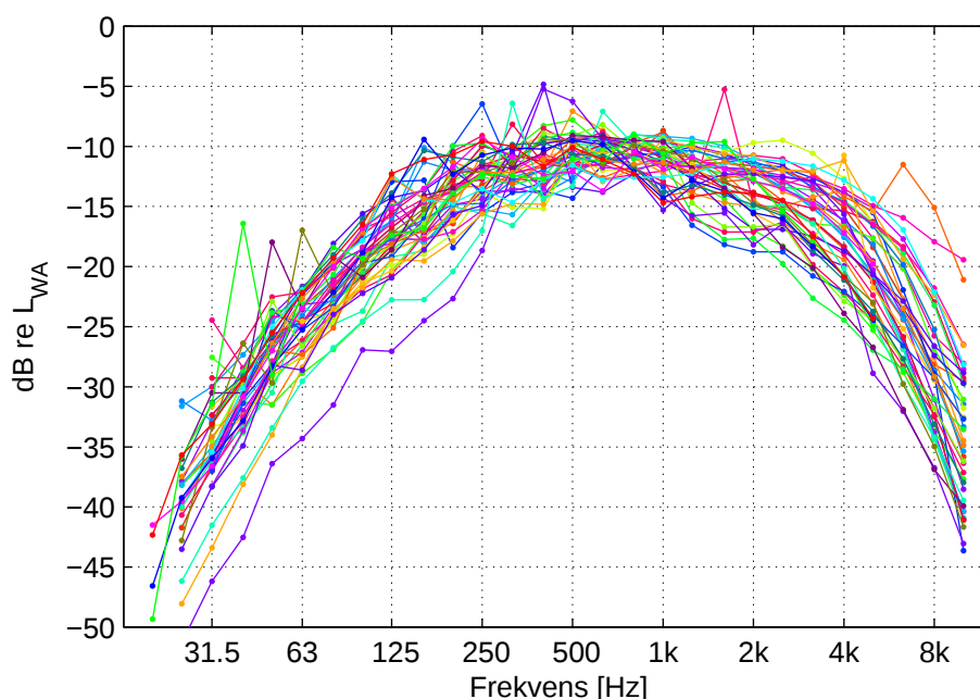
Figur 3. Normerede A-vægtede lydeffektniveauer i 1/3-oktavbånd. 45 møller med nominel elektrisk effekt mellem 75 kW og 3,6 MW. (Normeret svarer til, at L_{WA} for den individuelle mølle er trukket fra alle niveauerne i 1/3-oktavbånd).
