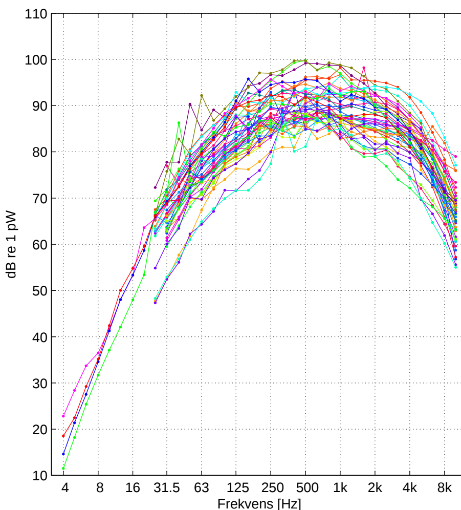
Figur 2. A-vægtede lydeffektniveauer i 1/3-oktavgbånd. 45 møller med nominal elektrisk effekt mellem 75 kW og 3,6 MW.
