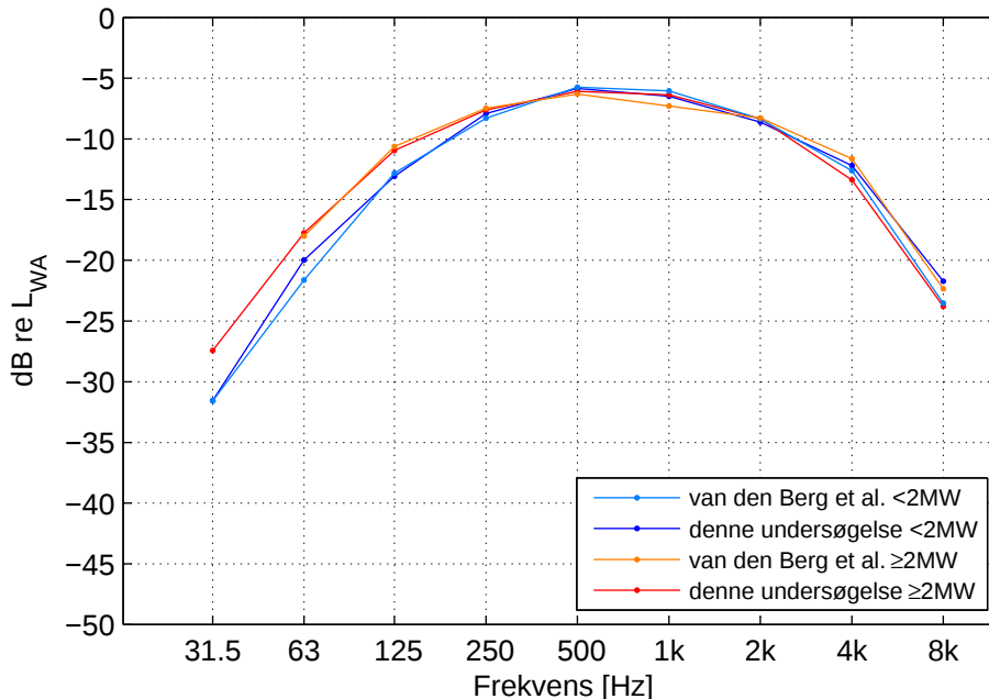
Figur 15. Normeret A-vægtet lydeffektniveau i oktavbånd, middelværdi af to grupper af møller: < 2 MW og ≥ 2 MW og fra to undersøgelser: van den Berg et al. [70, Appendix D] og denne undersøgelse.
