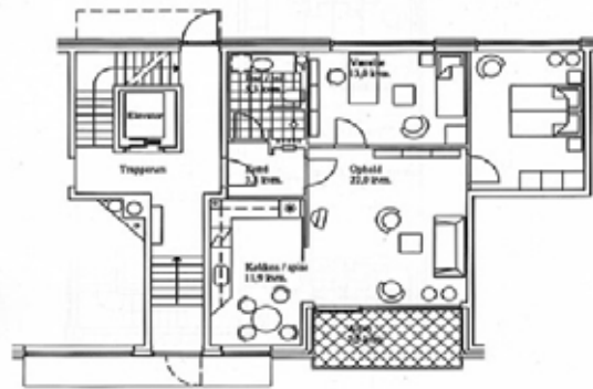
Type 2 st. 3-rums läjligt Bruttototal 91,9 kvm.
