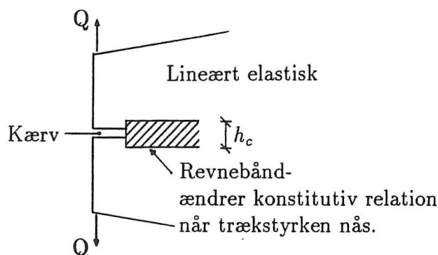
Figure 12: Betonemne påvirket til åbning, revnebåndmodellen
