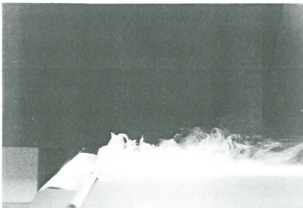
Figur 18. Aerodynamisk styret udsugning i bagvæg ved bord 5 sekunder efter, at en person er gået forbi bordet. V_u = 300 \text{ m}^3/\text{h} , v_i = 10 \text{ m/s} .
