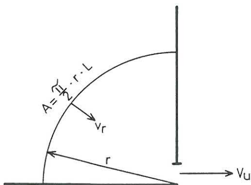
Figur 23. Principskitse af konventionel spalteformet udsugning mellem bord og bagvæg. r = afstand fra hjørne (m), v_r = hastighed (m/s) i afstanden r , A = areallet ( m^2 ) af en kvartcylinder med længden L (m) = bordets længde og V_u = udsuget luftmængde ( m^3/s ).
