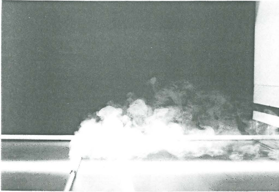
Figur 35. V_u = 400 \text{ m}^3/\text{h} , v_i = 10 \text{ m/s}
