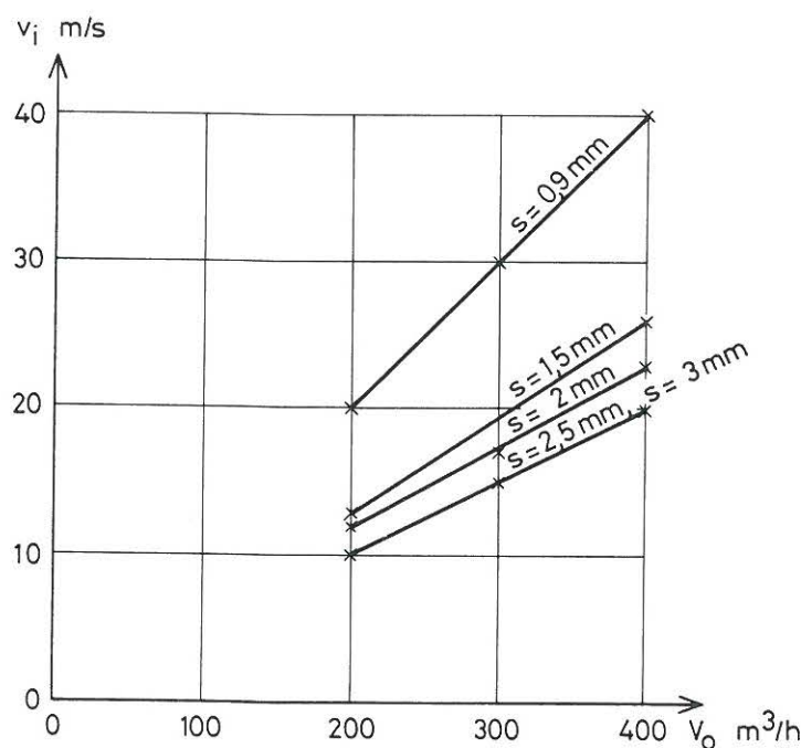
Figur 4. Kritisk indblæsningshastighed v_i som funktion af den udsugede luftmængde V_0 . Spaltehøjden s er parameter.
