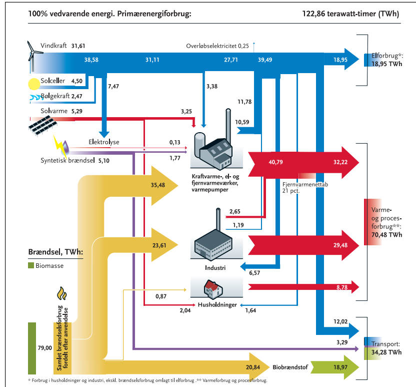
Figur 2. Energistrømme i 2050 i IDA's Klimaplan 2050.
