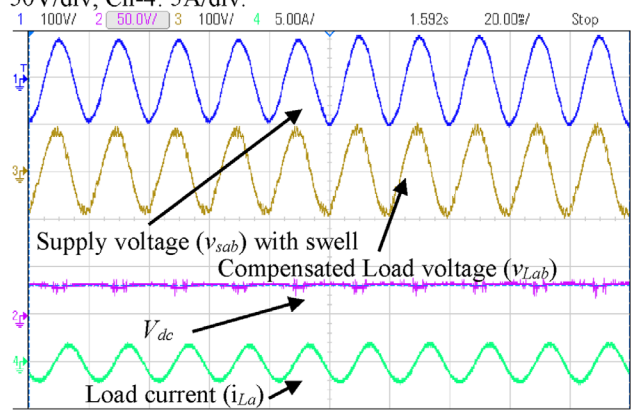
(d) X-axis- 50 \mu sec/div, Y-axis Ch-1,3: 100V/div, Ch-2: 50V/div, Ch-4: 5A/div.
