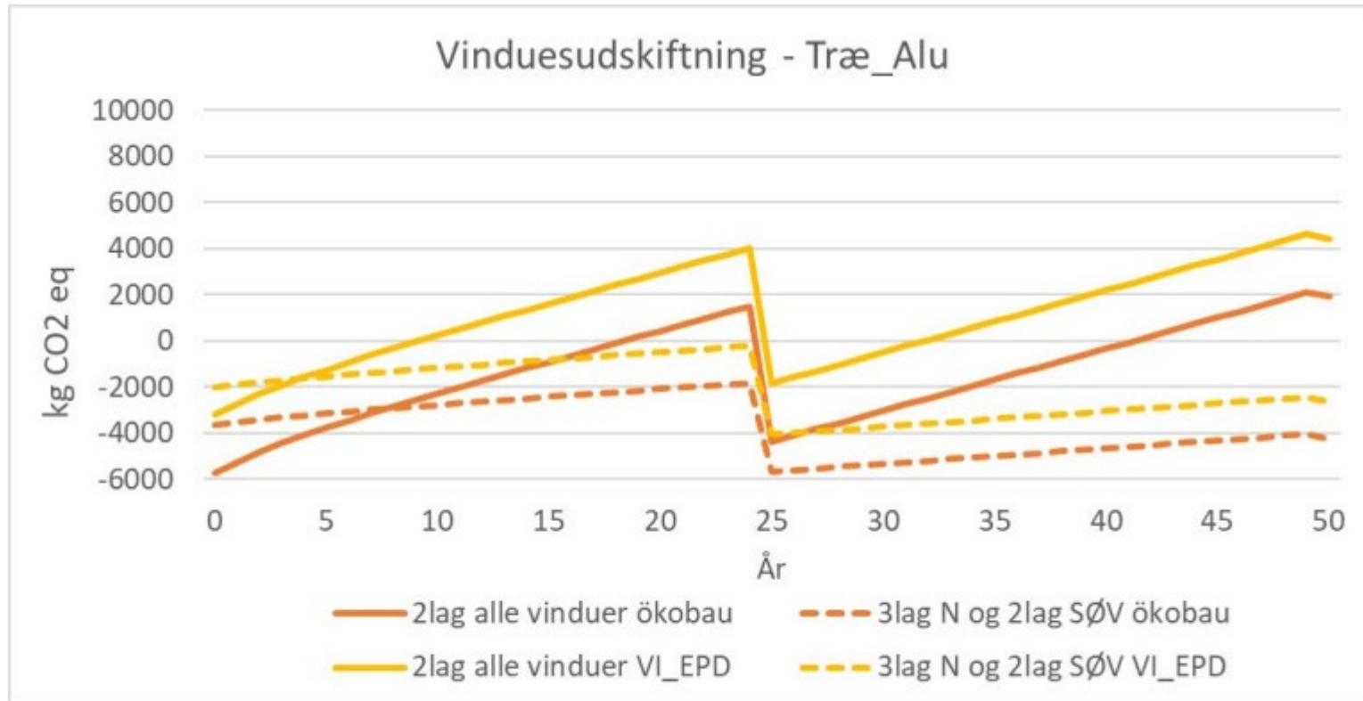
Figur 29. Etagebolig: Ændring i klimapåvirkning ved udskiftning af træ/alu vinduer til 2-lags vinduer og kombination af 2-lags- og 3-lags vinduer frem for 3-lags vinduer for hhv. økobau.dat data og gennemsnitsdata fra Vinduesindustrien.
