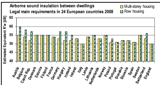
Figure 3 : Synthèse, pour 24 pays, des exigences minimales, exprimé en R'w équivalent (valeur parfois estimée), pour l'isolation au bruit aérien entre appartements, respectivement entre maisons mitoyennes. Tirée de [2].
