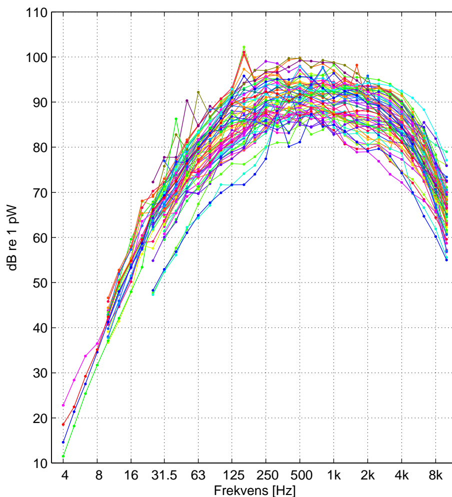
Figur 2. A-vægtede lydeffektniveauer i 1/3-oktavnånd. 62 møller med nominal elektrisk effekt mellem 75 kW og 3,6 MW.
