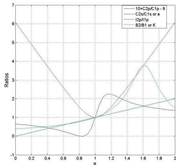
(d) K_s/K_p=2 , M/L_s=0.19 , Q=6
