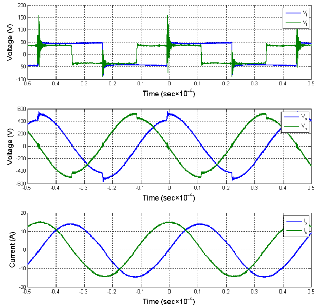
(d) Electrical quantities at Q_{13}
