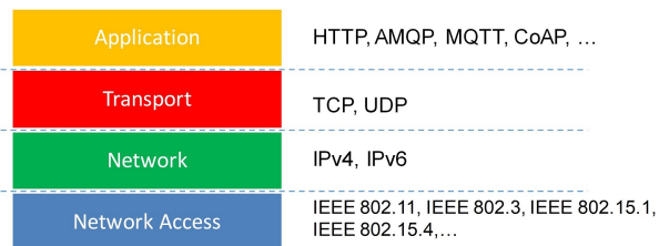
(b) IoT
