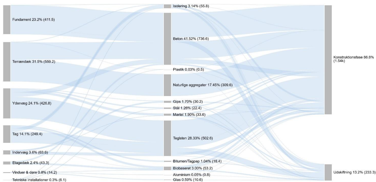
FIGUR 44. Materiale-mængder for enfamiliehus 1 for konventionel byggeskik (Enf,01) med en 100-årig betragtningsperiode for produktionsfasen og udskiftninger.
