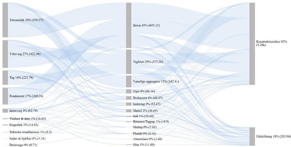
FIGUR 9. Materiale-mængder (kg/m 2 ) og materiale-mængdeandel (%) for konventionelt byggede enfamiliehuse fordelt på bygningsdele, materialekategorier, opførelse og udskiftning ved en 100-årig betragtningsperiode.
