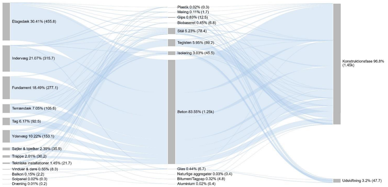
FIGUR 51. Materiale-mængder for etagebolig 2 for konventionel byggeskik (E k 02) med en 60-årig betragtningsperiode for produktionsfasen og udskiftninger.
