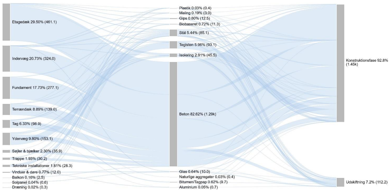
FIGUR 52. Materiale-mængder for etagebolig 2 for konventionel byggeskik (E k 02) med en 100-årig betragtningsperiode for produktionsfasen og udskiftninger.
