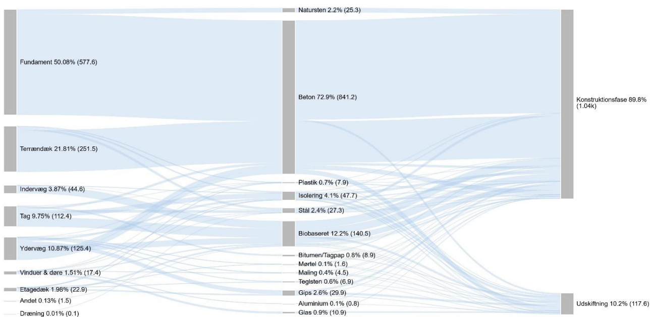
FIGUR 74. Materiale-mængder for kontorbygning 1 for træbaseret byggeskik (Kt01) med en 100-årig betragtningsperiode for produktionsfasen og udskiftninger.
