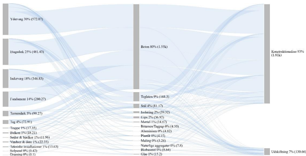
FIGUR 11. Materiemængder (kg/m 2 ) og materiemængdeandel (%) for konventionelt byggede etageboliger fordelt på bygningsdele, materialekategorier, opførelse og udskiftning ved en 100-årig betragtningsperiode.
