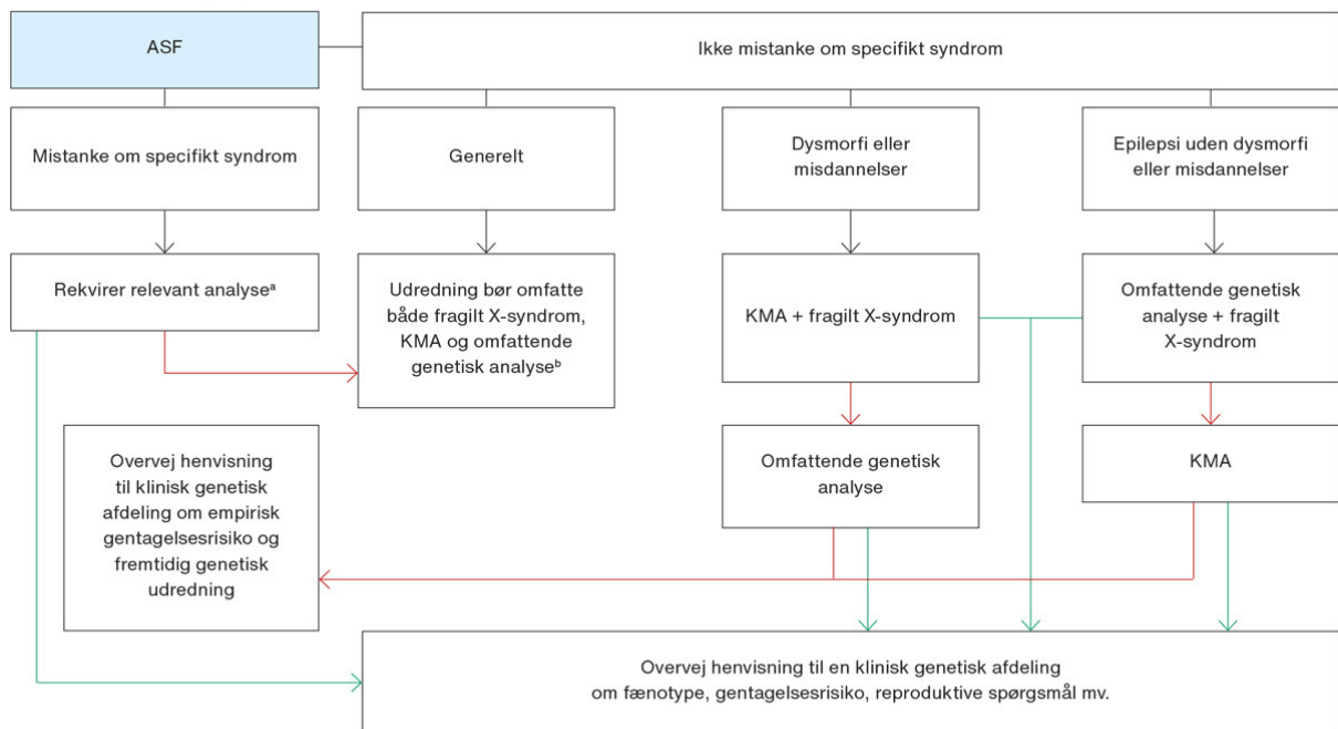
FIGUR 2 Udredningsalgoritme.
