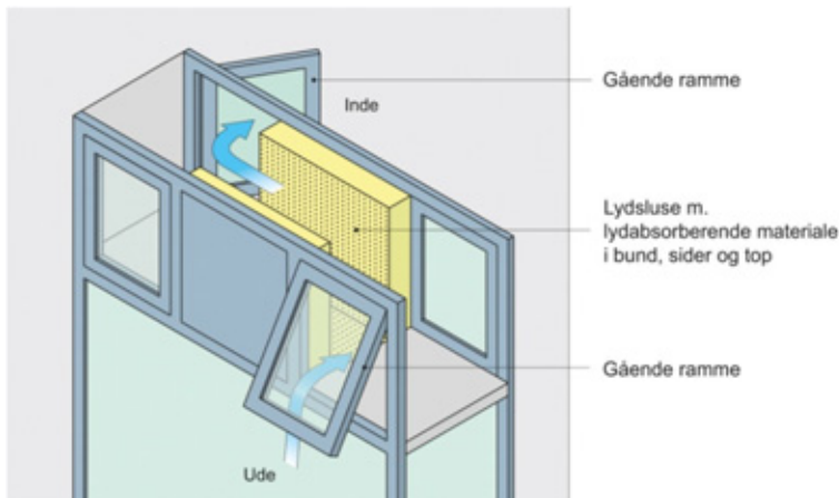
Figur 45. Eksempel på dobbelt vindueskonstruktion, hvor mellemrummene i de to vindueselementer er forbundet vandret via en lydsluse. For at opnå en god lydisololation skal udadgående og indadgående ramme åbnes diagonalt.
