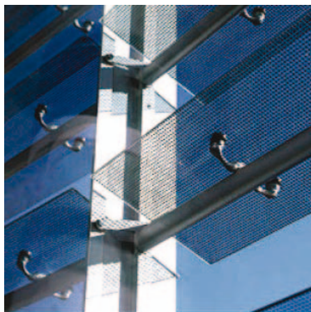
Figur 22. Glaslameller med integrerede solceller har været en attraktiv variant af bygningsintegrerede solceller hos mange arkitekter. Denne form for bygningsintegrering af solceller passer godt ind i tidens glasdominerende facadeudtryk, og løser samtidig behovet for en at anvende en effektiv udvendig solafskærmning (Blendex A/S).
