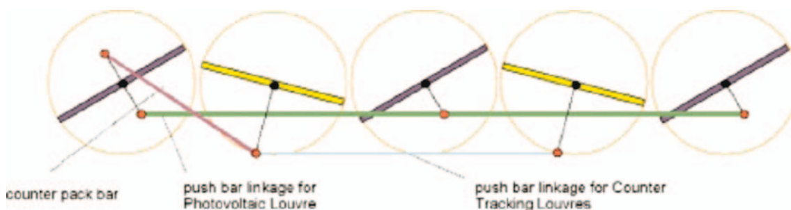
Figur 14. Eksempel på forsøg med at undgå indbyrdes skygger mellem lamellerne på afskærmninger med integrerede solceller. Hver anden lamel drejer lidt bort fra solen, hvorved der misteres en del i solintensitet og ydelse. Desuden vil afskærmningen næppe fungere optimalt som solafskærmning, der skal skærme af for solvarme og blænding.
