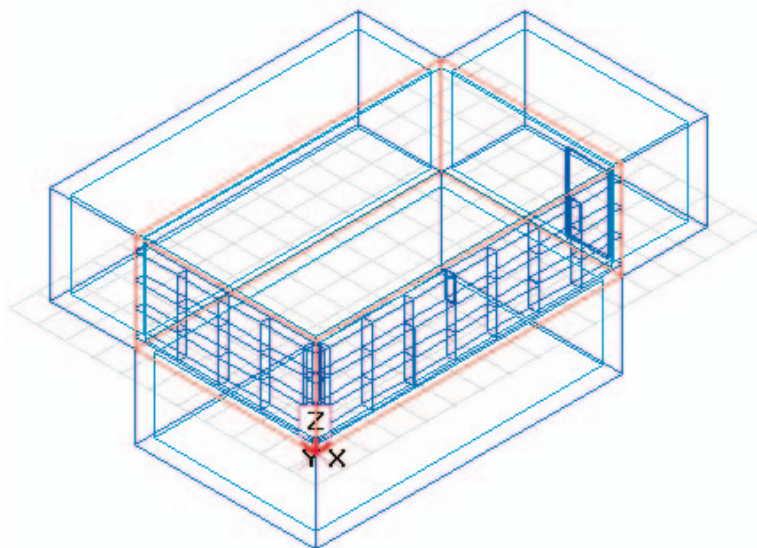
Figur 42. BSim-model for bygningen, der er simuleret som beskrevet i tabel 2 og tabel 3.
