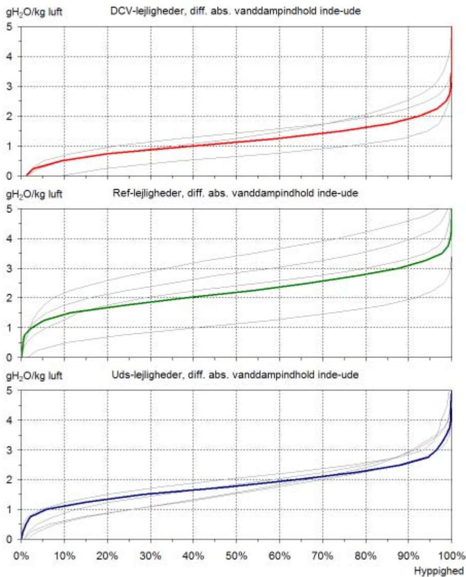
Figur 19. Figuren viser kumuleret, relativ fordeling af differensen mellem indeluftens og udeluftens absolute vanddampindhold i de tre grupper af lejligheder. Kurverne viser den procentvise andel af tiden i måleperioden, hvor differensen i vanddampindhold er lavere end angivet på ordinataksen. Abscisseaksen nederst er fælles for de tre diagrammer. De lysegrå kurver repræsenterer de enkelte lejligheder; de fuldt optrukne kurver angiver gennemsnittet for gruppen af lejligheder. Eksempel (rød kurve øverst): I gennemsnit for DCV-lejlighederne er differensen mellem indeluftens og udeluftens absolute vanddampindhold i 90 procent af tiden lavere end ca. 1,9 gH 2 O/kg luft.
