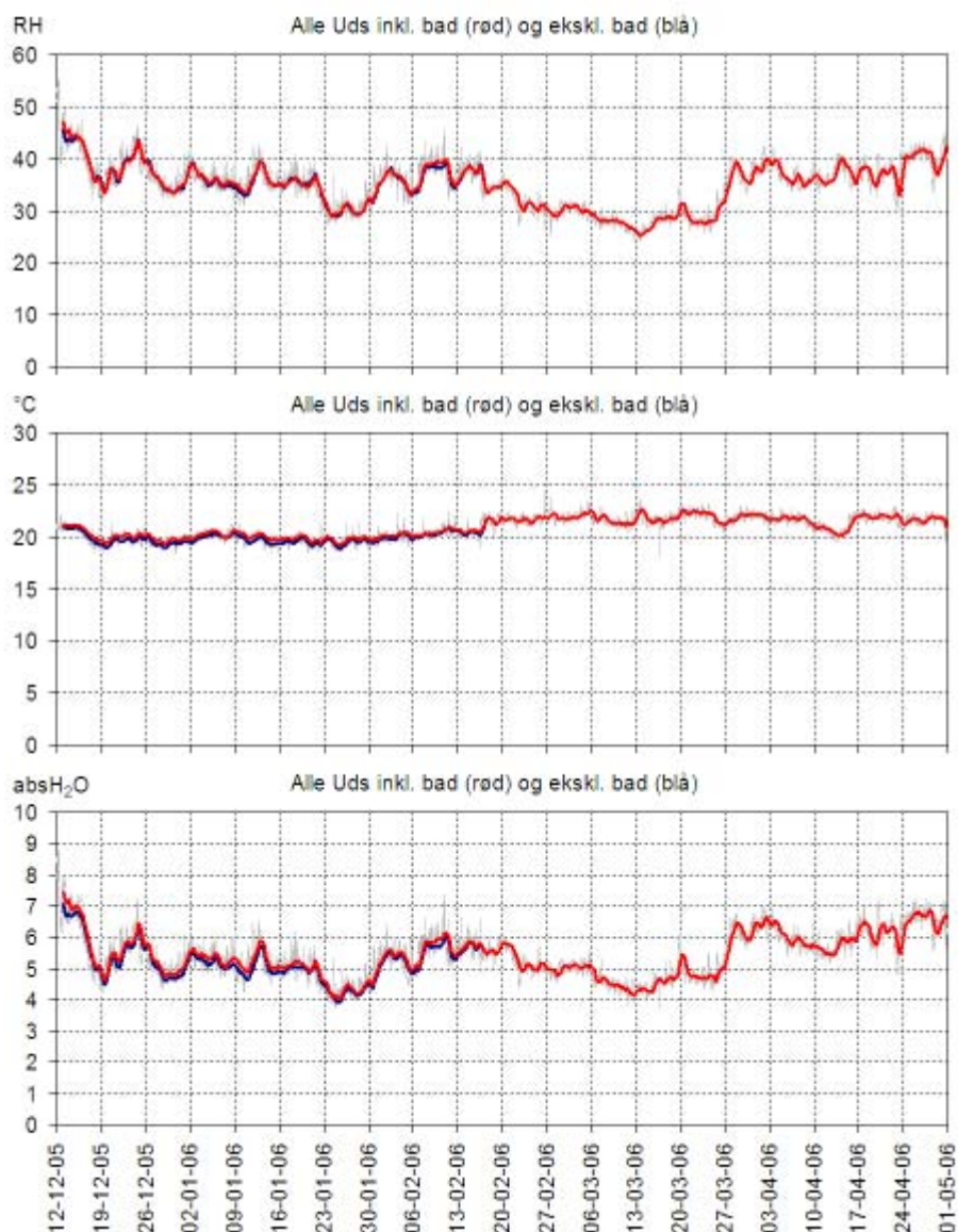
Figur 66. Figuren viser gennemsnittet for alle fire lejligheder med mekanisk udsugning af rumluftens relative fugtighed, rumtemperaturen og rumluftens absolute vandindhold henholdsvis eksklusive (blå kurve) og inklusive (rød kurve) måleresultaterne fra baderummet. De lysegrå kurver er 15 minutters registreringer; de fuldt optrukne kurver er døgnmiddelværdier.
