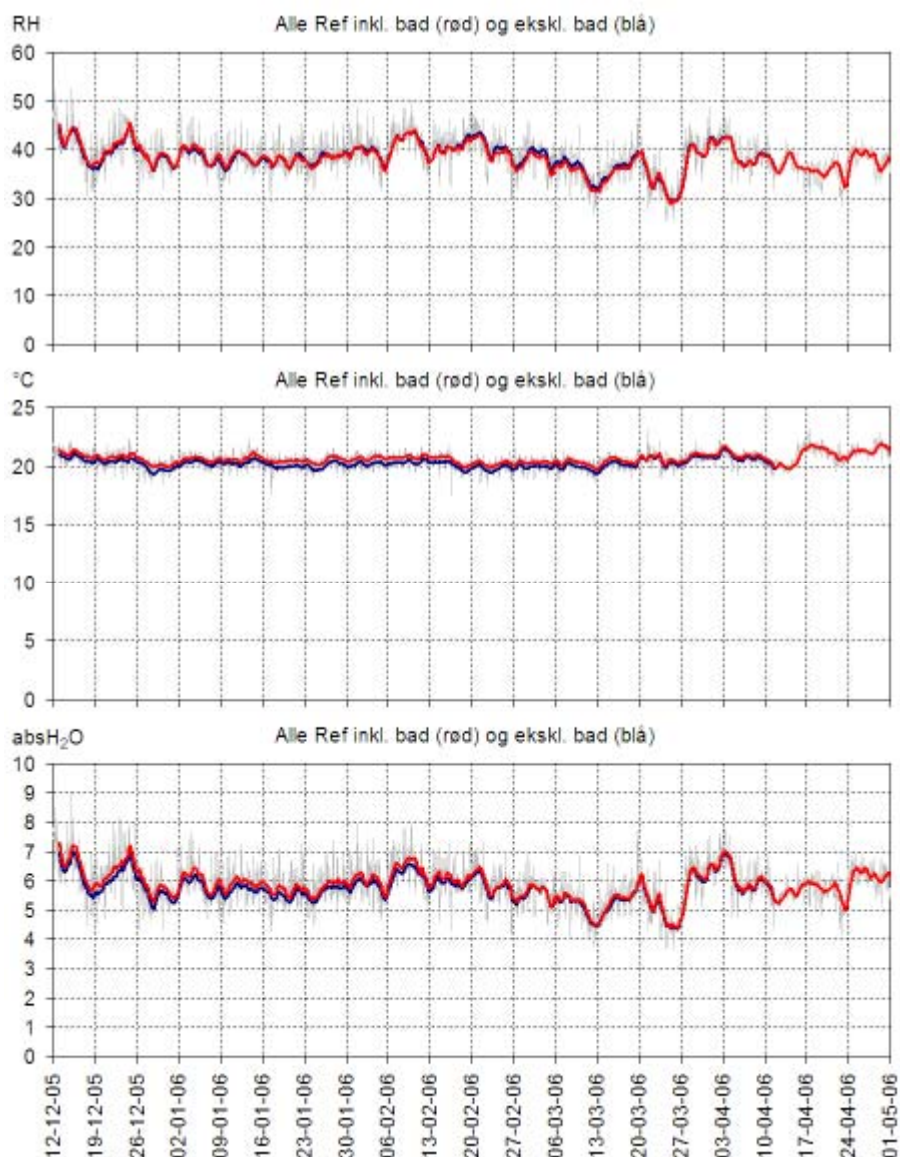
Figur 64. Figuren viser gennemsnittet for alle fire referencelejligheder af rumluftens relative fugtighed, rumtemperaturen og rumluftens absolute vandindhold henholdsvis eksklusive (blå kurve) og inklusive (rød kurve) måleresultaterne fra baderummet. De lysegrå kurver er 15 minutters registreringer; de fuldt optrukne kurver er døgnmiddelværdier.
