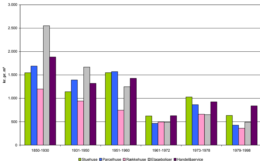
Figur 15. Omkostninger pr. m² opvarmet areal for forbedring af gennemsnitsbygningen i henhold til betingelserne i tabel 24.
