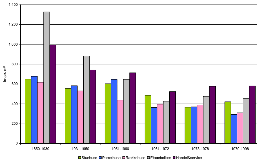
Figur 14. Omkostninger pr. m 2 opvarmet areal for forbedring af gennemsnitsbygningen i henhold til betingelserne i tabel 8.
