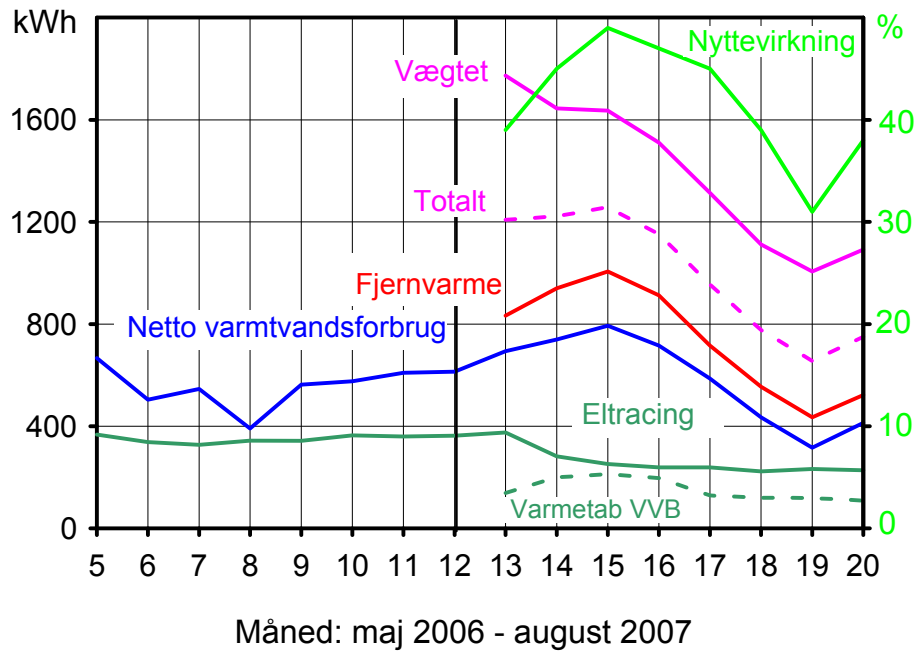
Figur B.2.17.5. Netto- og bruttoenergiforbrug, varmetab fra varmtvandsbeholder og eltracing samt nyttevirkning.
