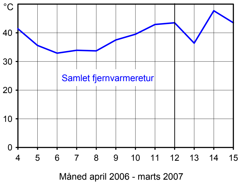
Figur B.2.12.6. Resulterende returtemperatur fra radiator- og brugsvandssystem.
