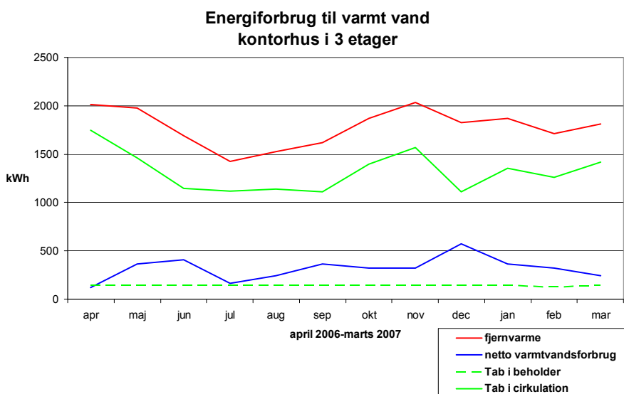
Figur B.2.7.4. Diagram over årsforbrug.
