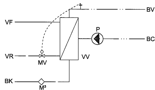
Figur 2.2.5. Varmtvandsproduktion, vekslerløsning.
