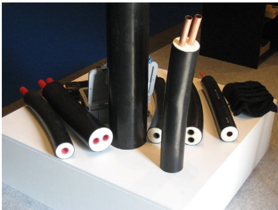
Figur 2.4.7. Præ-samisolerede rør.
