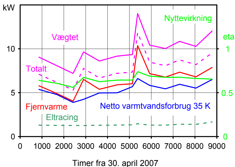
Figur B.2.22.5. Netto- og bruttoenergiforbrug samt eltracing og nyttevirkning. Ved den vægtede værdi er elforbruget ganget med faktor 2,5. Det beregnede nettovarmtvandsforbrug forudsætter en opvarmning af det kolde brugsvand på 35 K.
