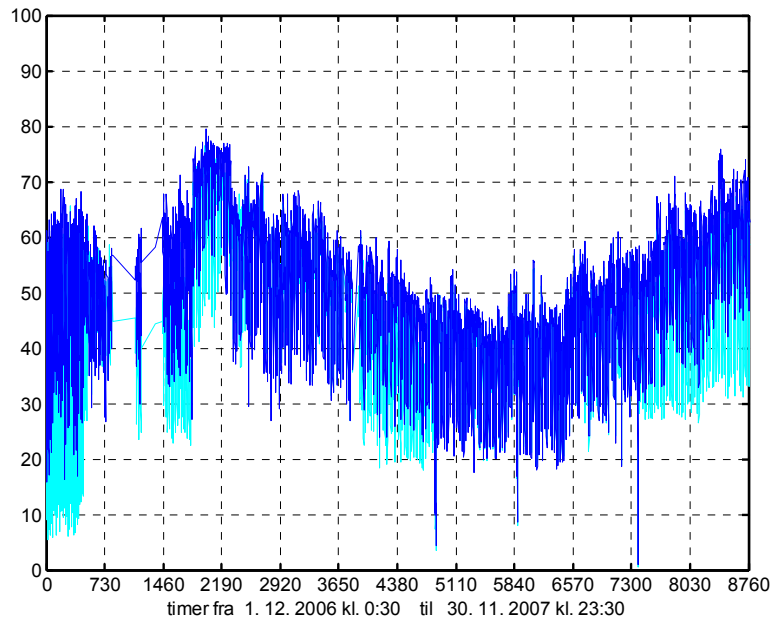
Figur B.2.13.8. Afkøling fra de to varmtvandsbeholdere.
