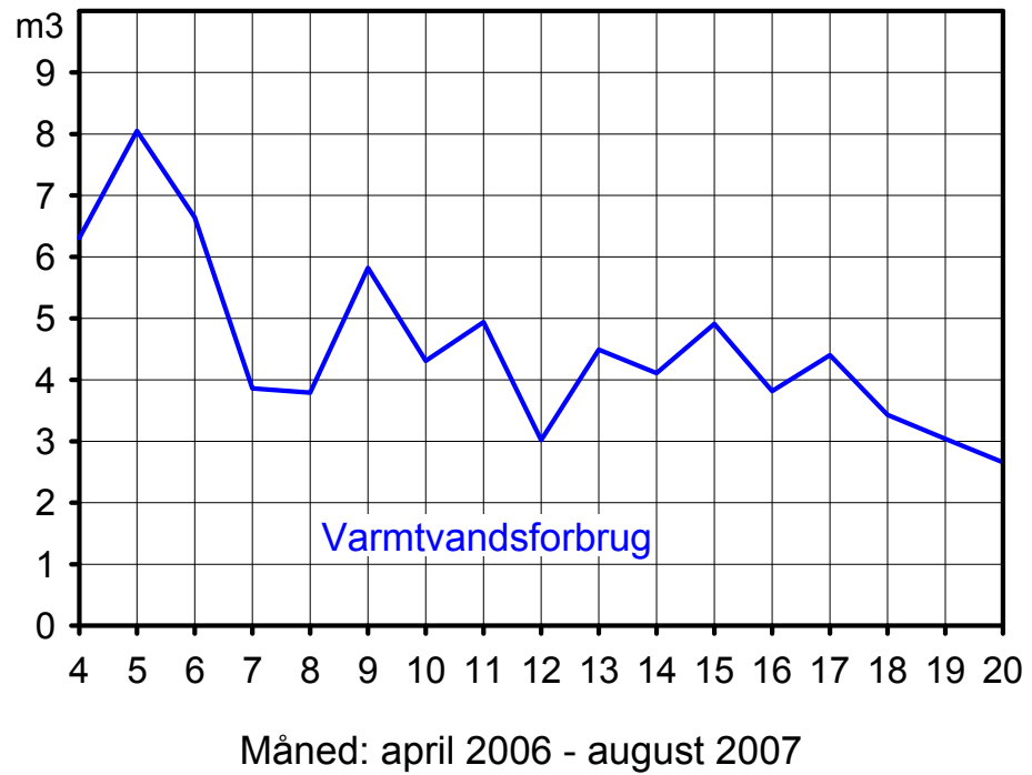
Figur B.2.15.4. Varmtvandsforbrug.
