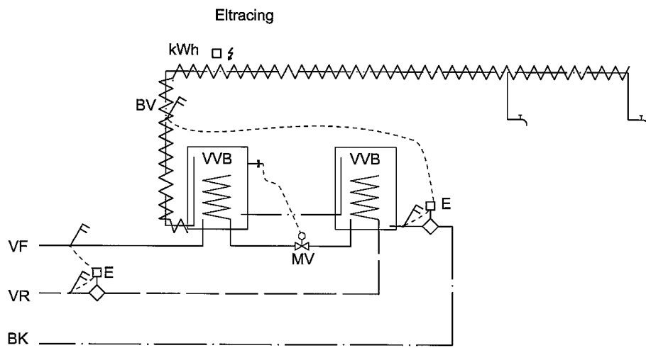
Figur B.2.17.2. Principdiagram.
