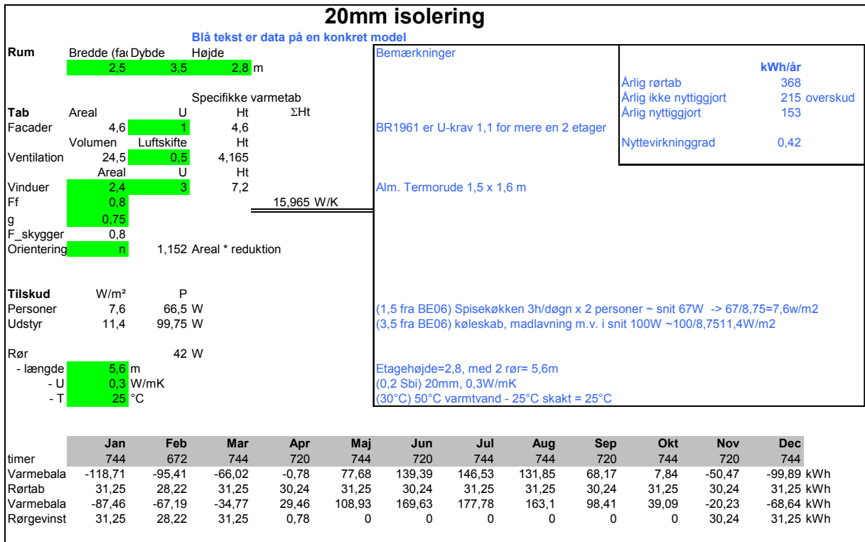
Figur 7.2.1. Eksempel på beregningsskema.
