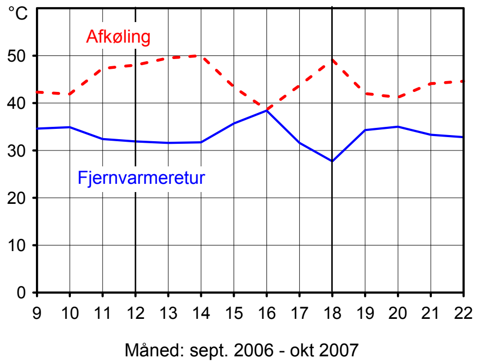
Figur B.2.18.6. Fjernvarmereturtemperatur og afkøling i brugsvandskredsen.
