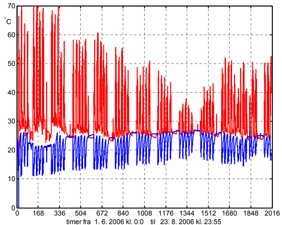
Figur B.2.14.11. Fremløbs- og returtemperaturer i varmtvandskredsen. Reguleringsventilens setpunkt er sat ned i løbet af perioden.
