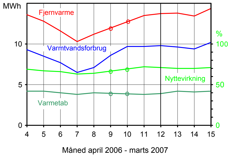
Figur B.2.12.5. Netto- og bruttoenergiforbrug, samt varmetab og nyttevirkning.
