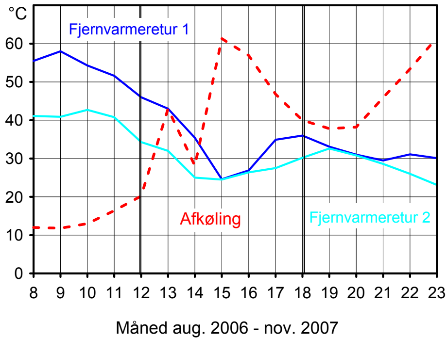
Figur B.2.13.6. Fjernvarmereturtemperatur fra de to varmtvandsbeholdere samt den fælles afkøling af fjernvarmevandet.
