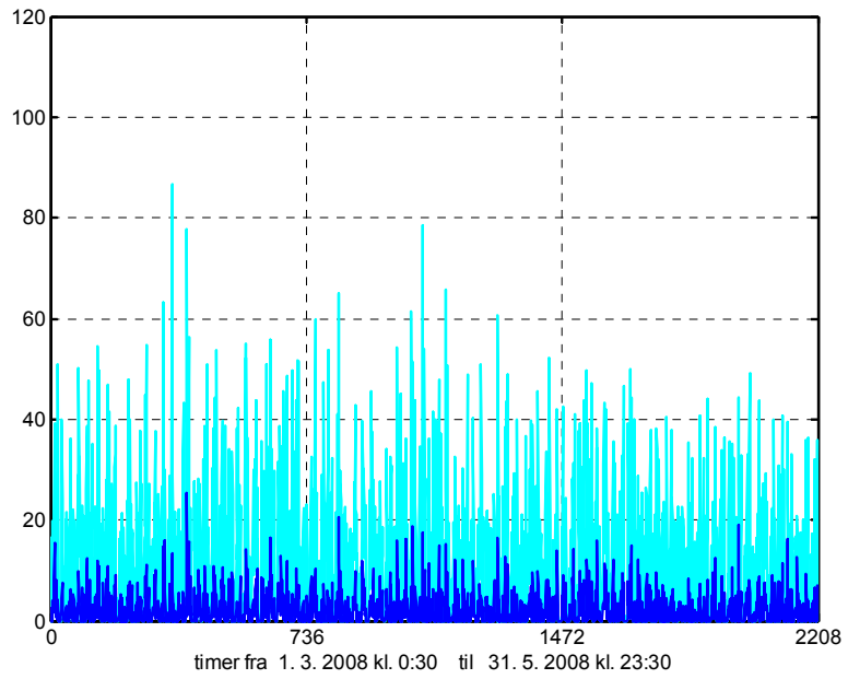
Figur B.3.1.10. Målt sekundær effekt på brugsvandssiden i kW. Mørkeblå: timeværdier, lyseblå: højeste 5-minutters værdi i hver time.
