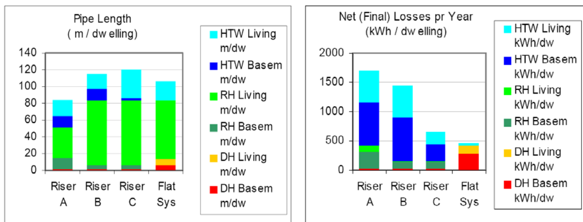
Figur 2.3.2. Sammenligning af ledningslængder pr. lejlighed, samt årligt nettovarmetab pr. lejlighed for 3 systemer med stigstreng og et system med fjernvarmefordeling til hver lejlighed. (Kristjansson, 2008).
