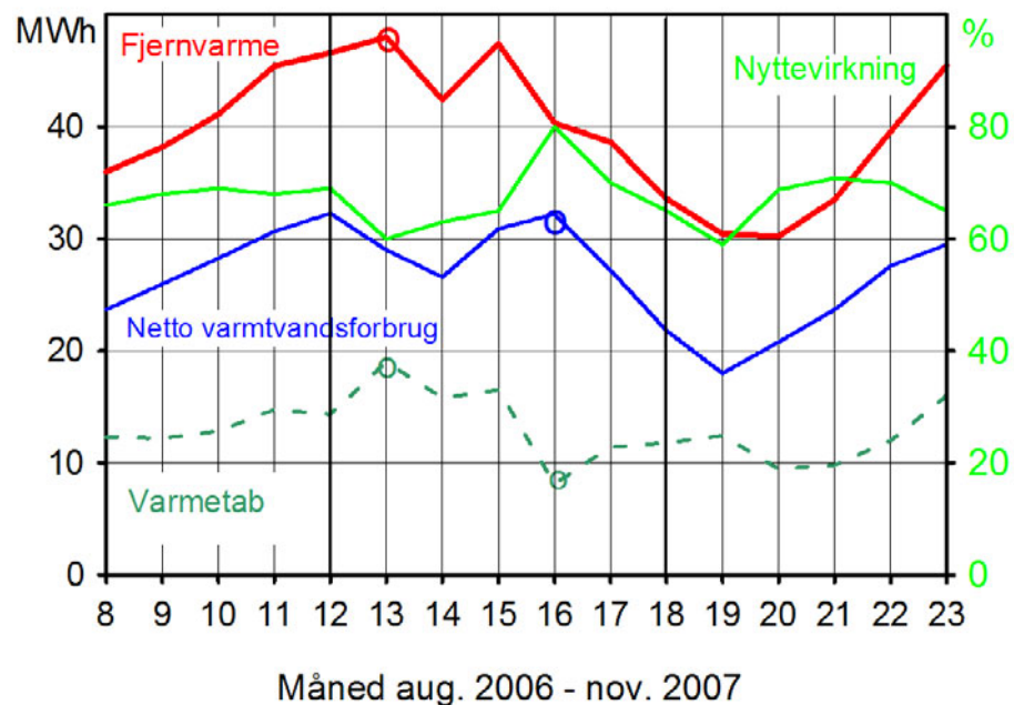
Figur B.2.13.5. Netto- og bruttoenergiforbrug samt varmetab og nyttevirkning.
