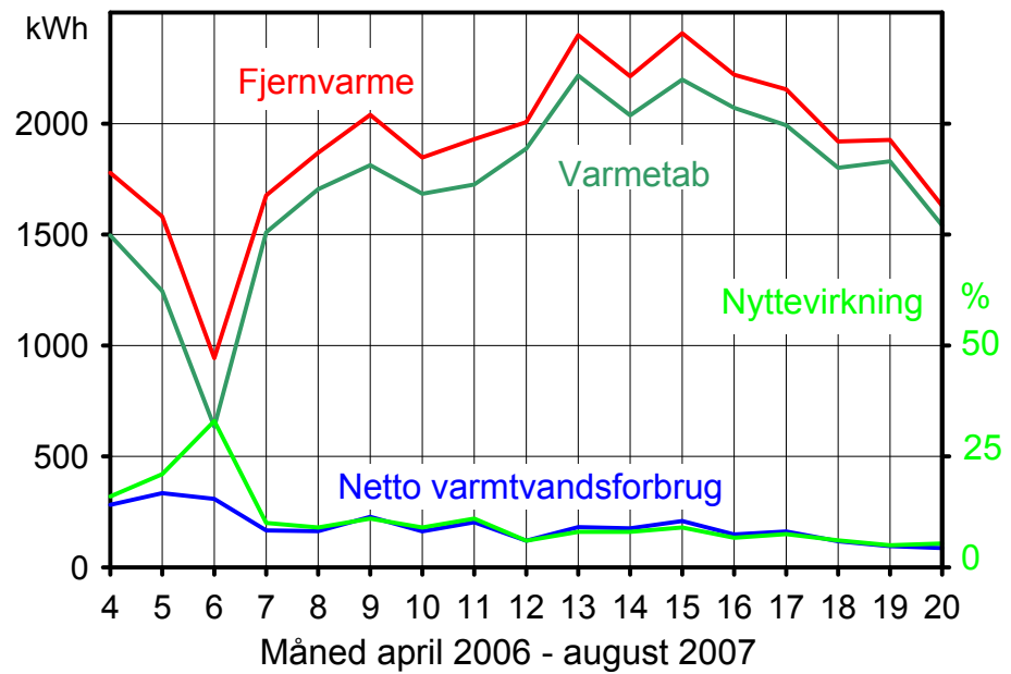
Figur B.2.15.5. Netto- og bruttoenergiforbrug samt varmetab og nyttevirkning.
