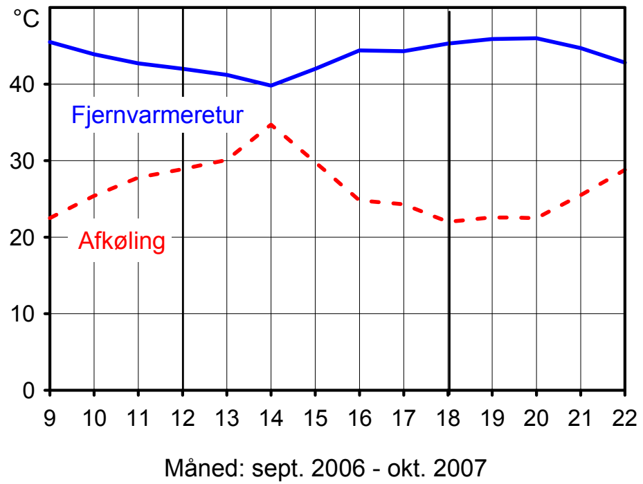
Figur B.2.19.6. Fjernvarmereturtemperatur og afkøling i brugsvandskredsen.
