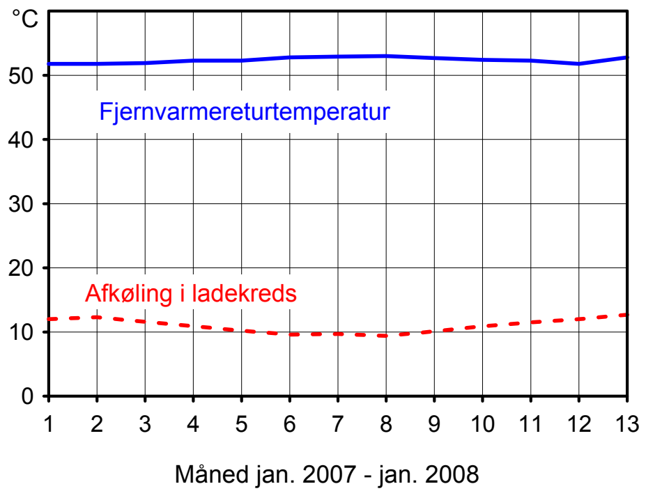
Figur B.2.20.6. Fjernvarmereturtemperatur og afkøling i shuntkredsen ved brugsvandsveksleren.
