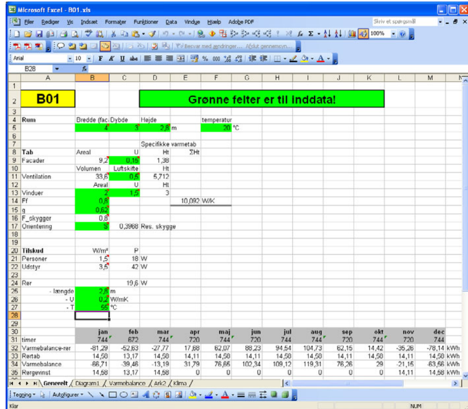
Figur B.4.1.2. Skærbillede fra beregningsmodellen for placering af rør til varmt vand gennem rum til beboelse.
