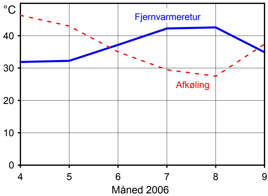
Figur B.2.11.6. Fjernvarmereturtemperatur og afkøling i brugsvandskredsen.
