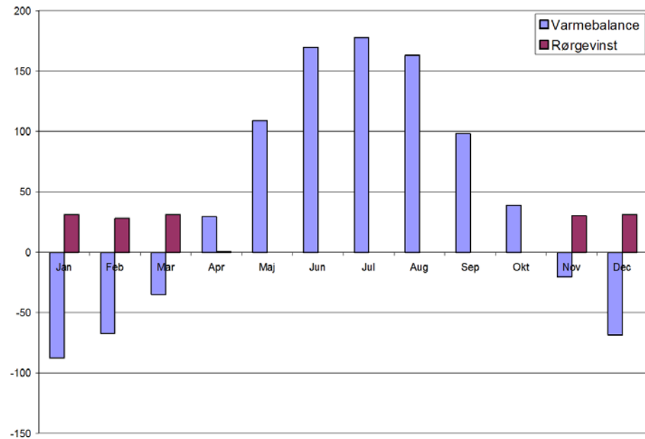
Figur 7.2.3. Eksempel på varmetab/varmetilskud i kWh pr. måned.
