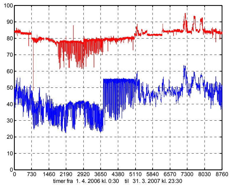
Figur B.2.12.9. Frem- og returtemperaturer til radiatorkredsen.
