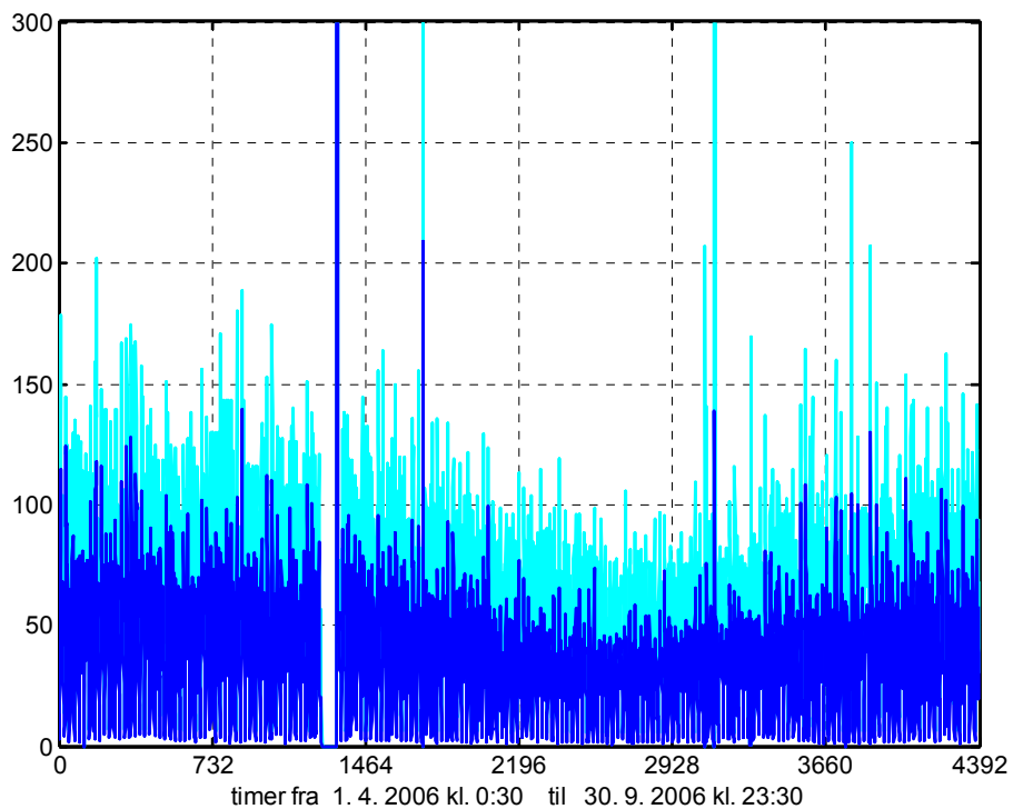
Figur B.2.11.10. Nettovarmtvandseffekt i kW (beregnet ud fra flowpulser og temperaturer); mørkeblå: timeværdier, lyseblå: højeste 5-minutters værdi i hver time.
