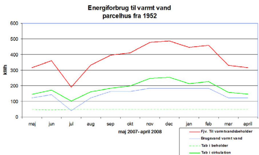
Figur B.2.9.4. Diagram over årsforbrug.
