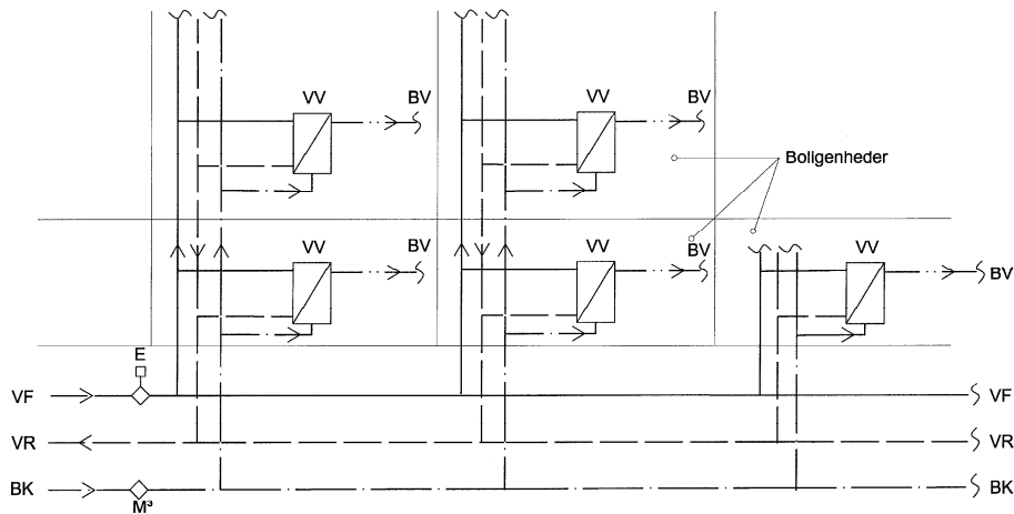
Figur 2.2.3. Decentral varmtvandsproduktion.
