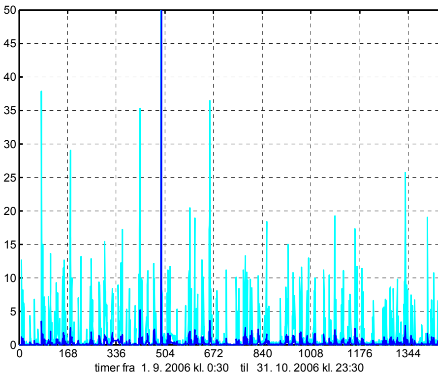
Figur B.2.15.10. Nettovarmtvande-effekt i kW. Mørkeblå: timeværdier, lyseblå: højeste 5-minutters værdi i hver time.
