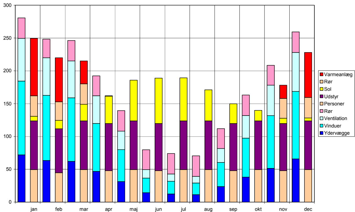
Figur 7.2.2. Eksempel på varmebalance/rørgevinst i kWh pr. måned.
