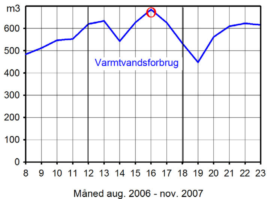
Figur B.2.13.4. Varmtvandsforbrug.
