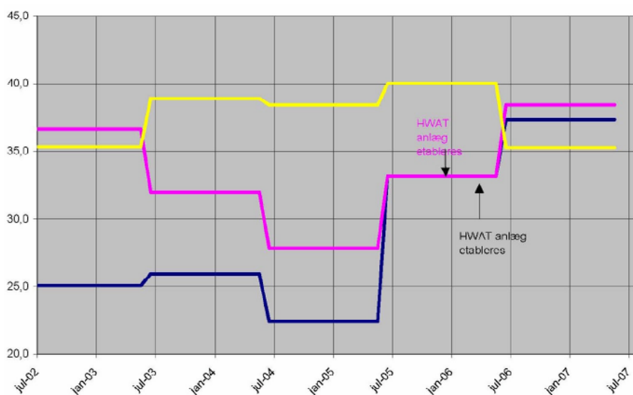
Figur 2.5.1. Afkøling i tre boligejendomme, hvoraf de to har udskiftet cirkulationssystemet med eltracing, Lund (2008). Gul kurve: Ejendom A, cirkulation. Violet kurve: Ejendom B, eltracing. Blå kurve: Ejendom C, eltracing.
