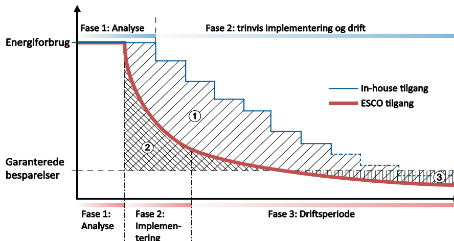
Figur 1. Den principielle forskel på ESCO-indsats (nederst, rød farve) og en in-house energirenovering (øverst, blå farve) der foregår trinvist over en årrække. Forskellen mellem de to metoder udgøres af område 1, 2 og 3 tilsammen.
