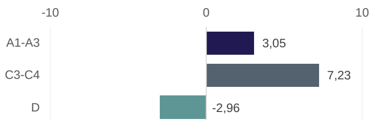
Figur 31 Klimapåvirkning i kg CO 2 -eq pr. m 2 tagpap for henholdsvis produktionsfasen (A1-A3), bortskaffelsesfasen (C3-C4) samt potentialet ved genanvendelse (D)
