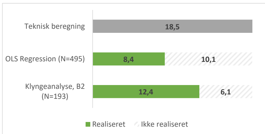
Figur 3.4. Estimat for teknisk beregning sammenlignet med estimater for reelle forskelle i varmeforbrug (kWh/m 2 ) (her realiseret) med og uden efterisoleret loft for gruppe B (1962 til 1978).
