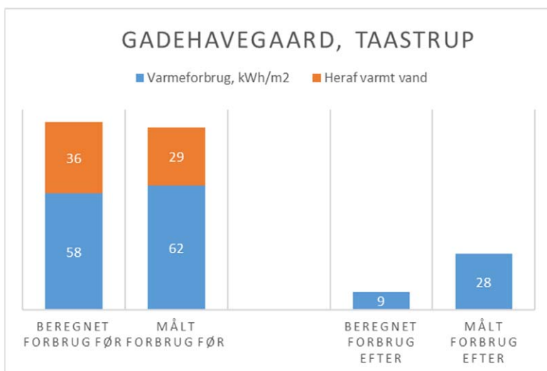
Figur 4.3. Beregnede og reelle varmekonsum i Gadehavegaard, før og efter renovering. Kilde: TI (2018)
