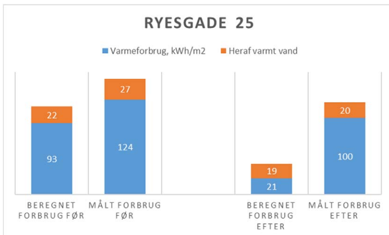
Figur 4.2. Beregnede og reelle varmekonsumtion i Ryesgade 25, før og efter renovering. Kilde: (Teknologisk Institut, 2018).
