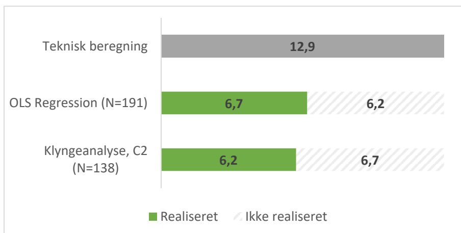
Figur 3.5. Estimat for teknisk beregning sammenlignet med estimater for reelle forskelle i varmeforbrug (kWh/m 2 ) (her realiseret) med og uden efterisoleret loft for gruppe C (1979 til 1999).
