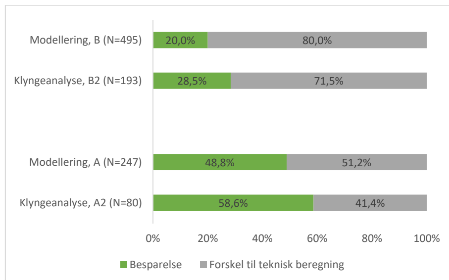
Figur 3.6. Sammenligning af forskellen i varmekonsum i forhold til den tekniske beregnings estimat for nye vinduer i procentandel.
