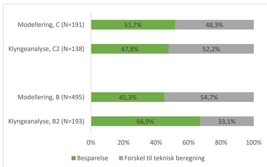
Figur 3.7. Sammenligning af forskellen i varmekonsum i forhold til den tekniske beregnings estimat for efterisolering af loft i procentandel.
