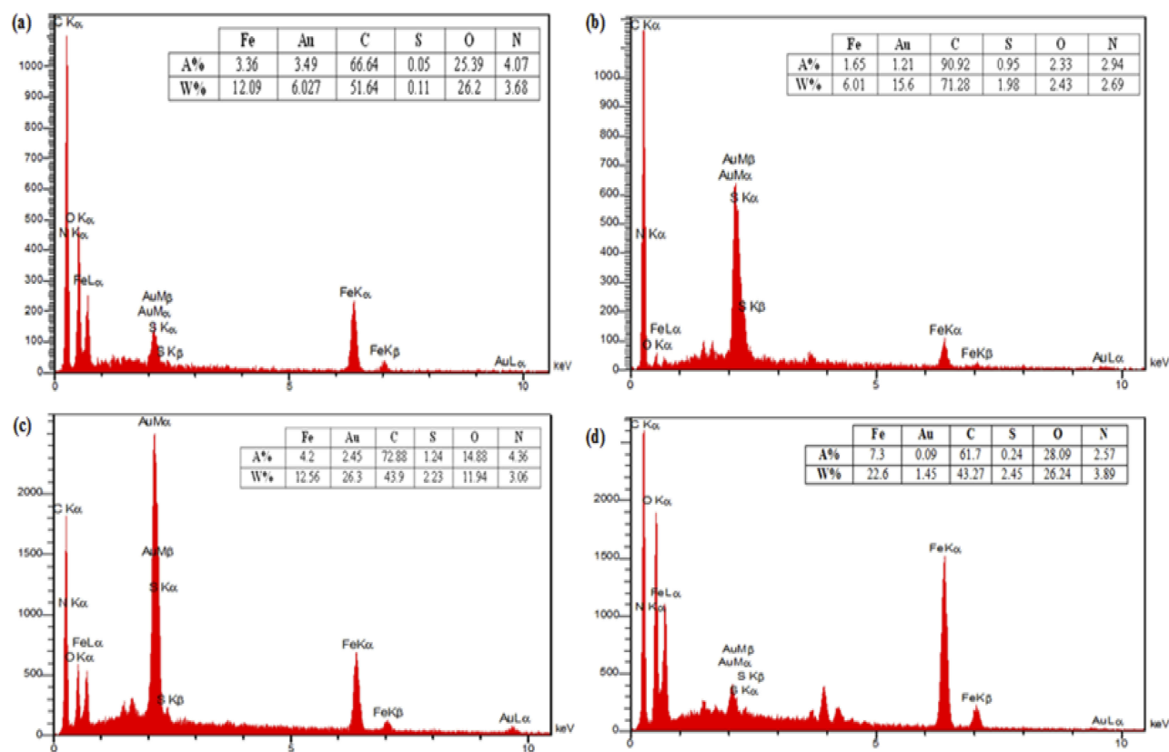
Figure 8 EDX analysis of (A) \gamma -Fe 2 O 3 @Au/PβCD, (B) \gamma -Fe 2 O 3 @Au/PβCD/PAA-SDN, (C) \gamma -Fe 2 O 3 @Au/PβCD/PAA-SDN/PEI-βCD and (D) Nanocapsule.
