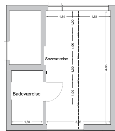
Figur 2-10 – Skitse af målepunkterne på centerlinjen i midten af rummet
