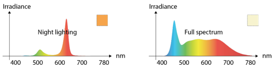
Figur 3-1 - Principiel skitsering af LED-spektralfordelingen (SPD) for de testede lys-scenarier. På venstre side et belysningsscenario uden korte (blå) bølgelængder og på højre side et fuldspektrum belysningsscenario
