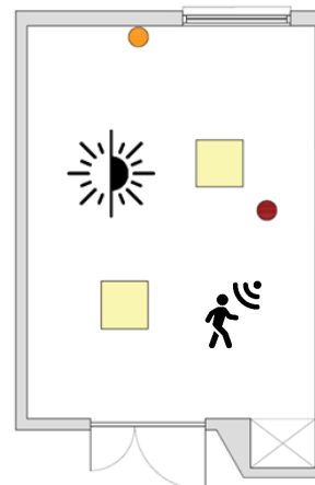
Figur 4-9 Det eksisterende belysningsystem med to LED-armaturer, en wallwasher og en læselampe ved sengen med et dagslysafhængigt kontrolsystem
