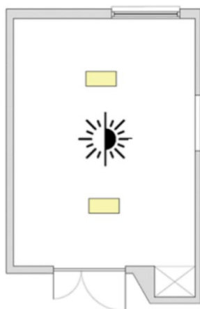
Figur 4-7 Standardbelysningsystemet med to LED-paneler placeret i sengestuen reguleret ud fra dagslyset (der opnås nok belysningsstyrke på 300 lux om dagen ved 2 LED-paneler, derfor ændret i forhold til de andre cases.
