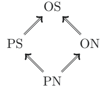
Fig. 3: Hierarchy
