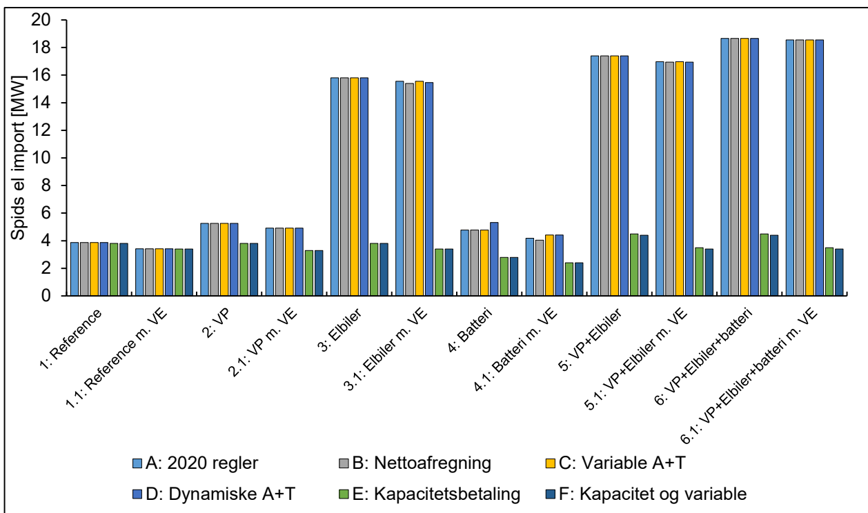
Figur 30 – Årlig spidsimport af el fra elnettet til energifællesskabet i hvert scenarie.
