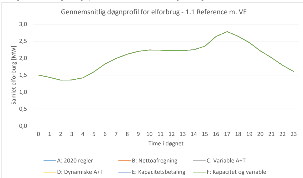
Figur 7 – Gennemsnitlig døgnprofil for elforbrug i 1.1 Reference m. VE scenarierne.
