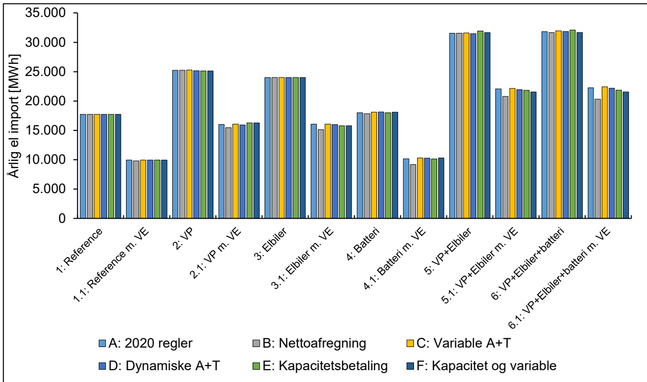
Figur 31 – Årlig import af el fra elnettet til energifællesskabet i hvert scenarie.
