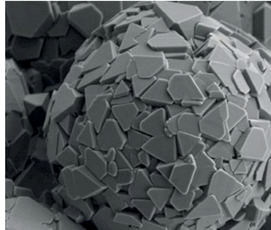
Figur 11: Visualisering af LMNO-partikler vha. scanningselektron-mikroskopi. De tætte runde partikler er udviklet for at kunne opnå høj energitæthed i LNMO-batterierne.
