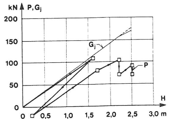
Fig. 11. Variation af jordlasten på målerør 1 angivet som den prøvningslast, P, der fremkalder samme værdi af deformationen \gamma_c . Til sammenligning er vist referencelasten G_j . H er fyldhøjden over rørtop.
