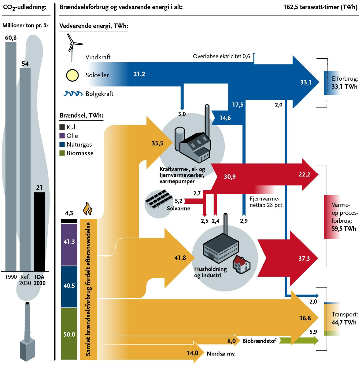
Figur 2.2: Energistrømme i referencen for år 2030 og for IDAs Energiplan 2030.
