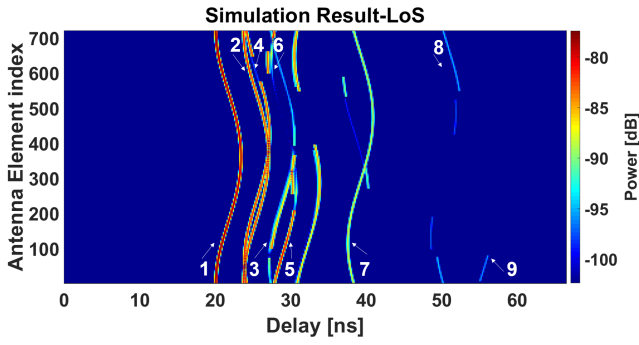
Fig. 8. Simulated CIR in LoS scenario.
