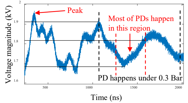
Fig. 22. PD region under 0.3 Bar
