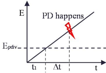
Fig. 20. PD time lag
