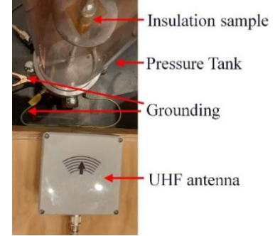
Fig. 9. UHF antenna
