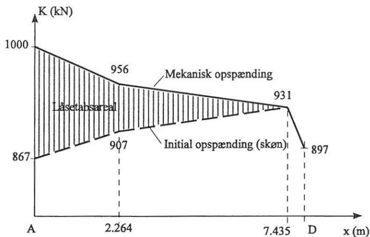
Figur 4. Kraftdiagram
