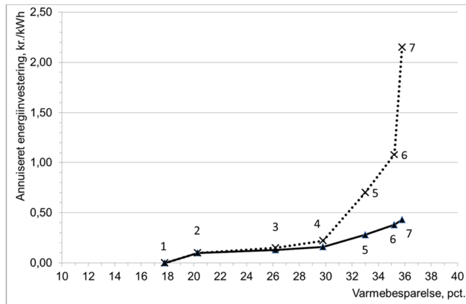
Figur 1 Annueret energiinvestering i kr./kWh i afhængighed af varmesparelsen i pct. Optrukket kurve er summeret investering for scenarierne og stiplede kurve er marginal investering for det sidste scenarie. Tal på kurve er scenarienummer.
