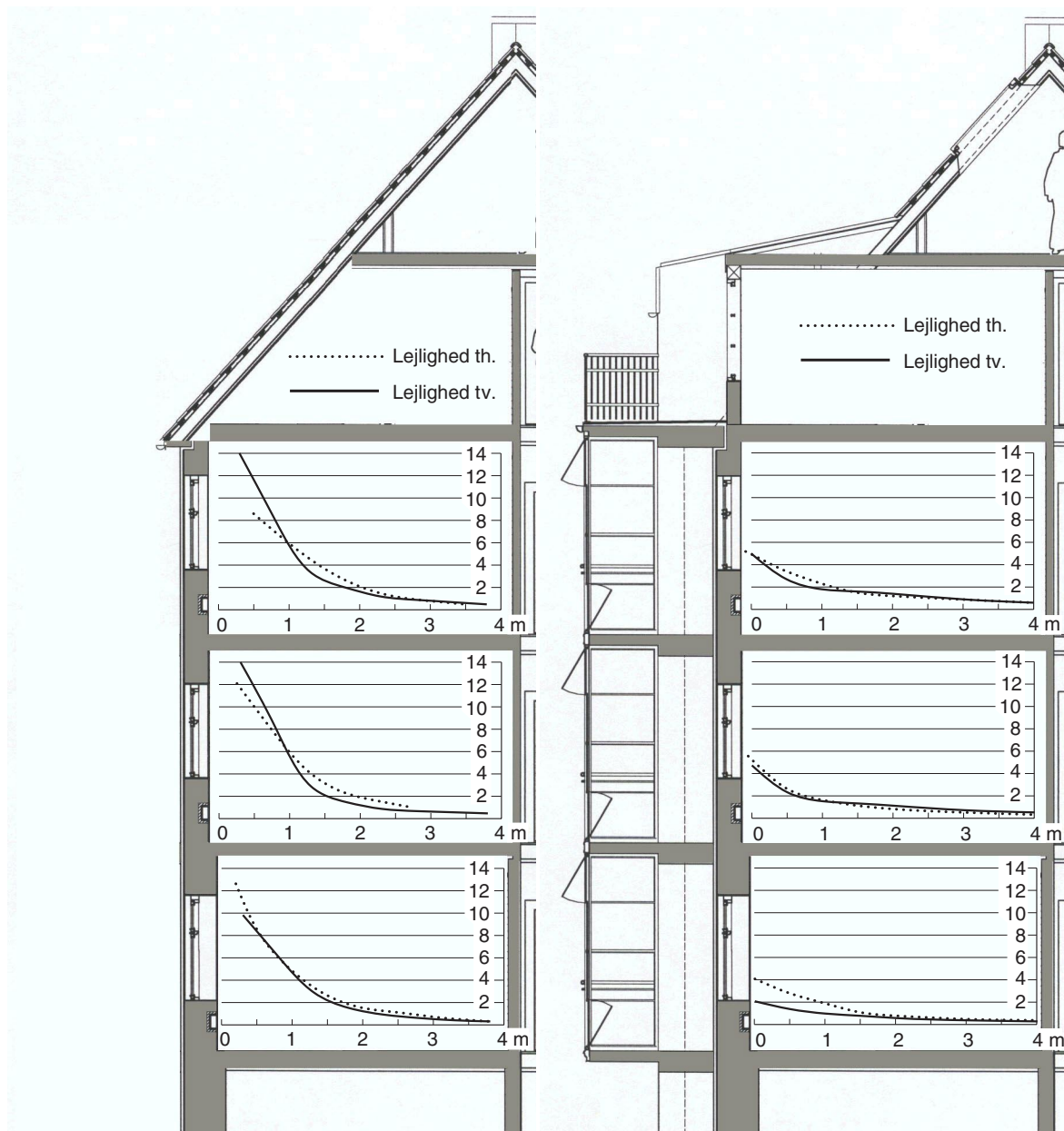
Dagslysforskelene før og efter renoveringen. Tilbygningen reducerer permanent dagslysniveauet mest lige inden for vinduet (ca. 75 %) og mindre bag i rummet (ca. 25 % midt i). De højere dagslysfaktorer i lejlighederne til venstre (efter renovering) skyldes det nye vindue i gavl.
