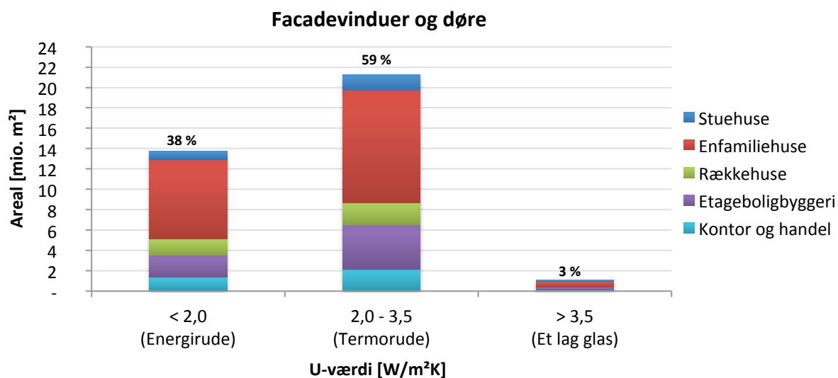
Figur 44. Opskaleret vindues- og dørareal ud fra energimærkningsdatabasen og BBRregistreringen. Vinduer med ét lag glas antages at have en U-værdi større end 3,5 W/m²K, vinduer med termoruder (el. to separate glas) antages at have en U-værdi mellem 2,0 og 3,5 W/m²K, og nyere vinduer med energiruder antages at have en U-værdi mindre end 2,0 W/m²K.
