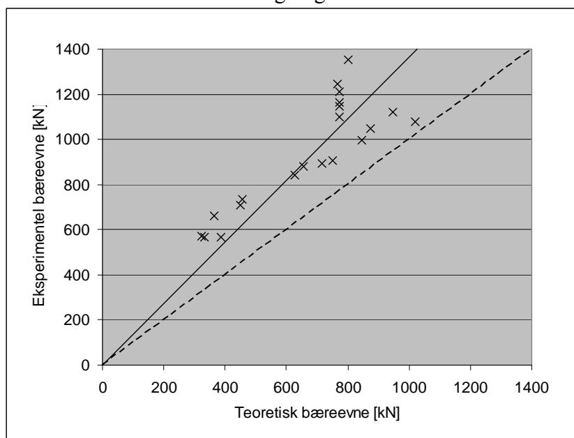
Figur 4.1. Sammenhørende værdier af eksperimentel bæreevne N_{test} og bæreevne efter DS411:1998, N_{teori} markeret med x. Fuldt optrukket linie: bedste fit med statistisk model i aneks A. Stiplet line: eksperimentel bæreevne lig beregnet bæreevne.
